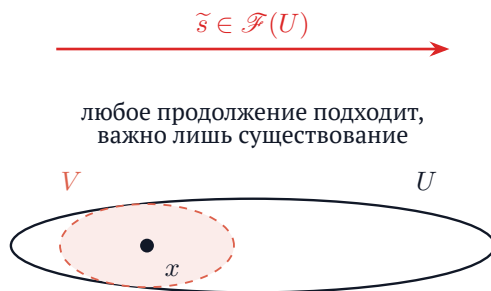
Рис. 12.1. Фласковость: сечение над V \subset U обязательно продолжается до сечения над U (красная стрелка — любое такое продолжение; нулевое продолжение тоже годится).
