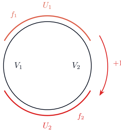
Рис. 3.3. Окружность: классы f_1 и f_2 согласованы в \mathcal{P} , но глобального сечения нет (Манин, рис. 2.2).
