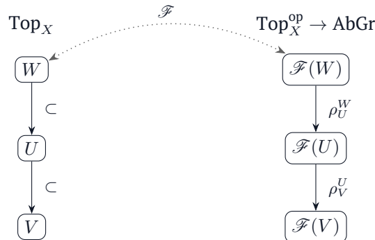
Рис. 3.1. Контравариантный функтор: морфизмы \text{Top}_X идут в ту же сторону, а значения предпучка — в противоположную. Поэтому ограничение \rho_U^V переводит сечение с большого открытого множества на меньшее .
