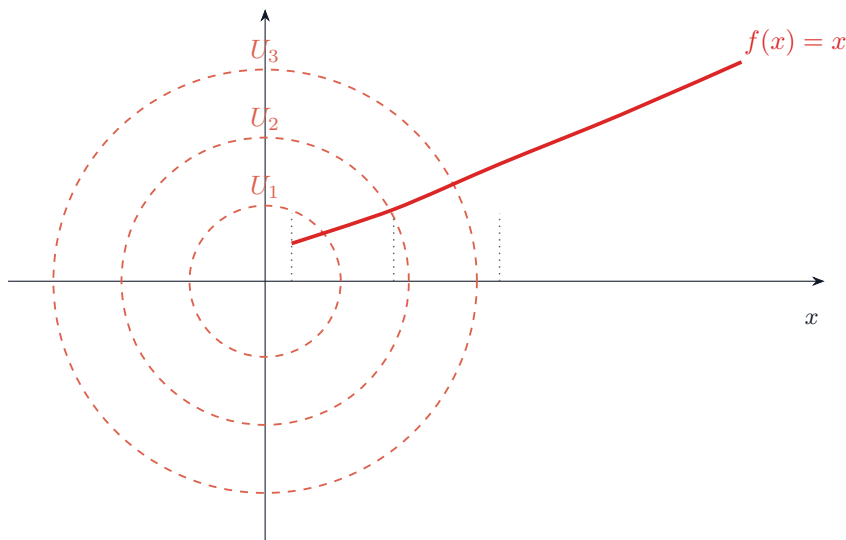
Рис. 3.4. Нарушение (F2) для ограниченных функций: локальные сечения согласованы и покрывают \mathbb{R} , но их склейка не ограничена.
