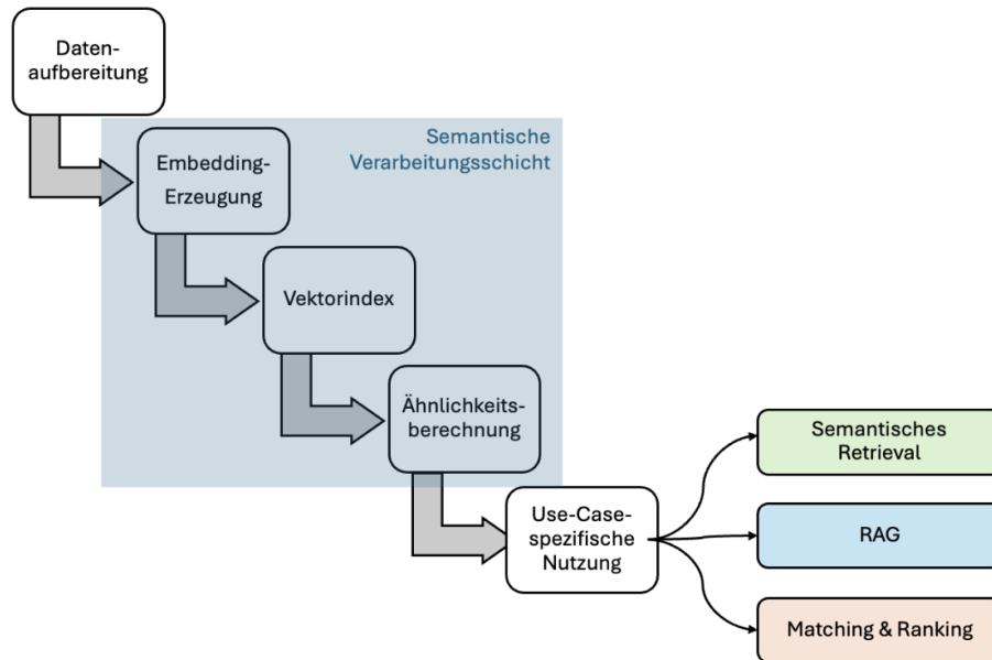
Abbildung 6: Grundarchitektur der Verarbeitung Embedding-basierter Systeme.
