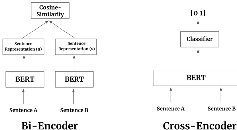
Abbildung 4: Schematische Gegenüberstellung von Bi-Encoder- und Cross-Encoder-Architekturen anhand von BERT Soliman (2022) .
