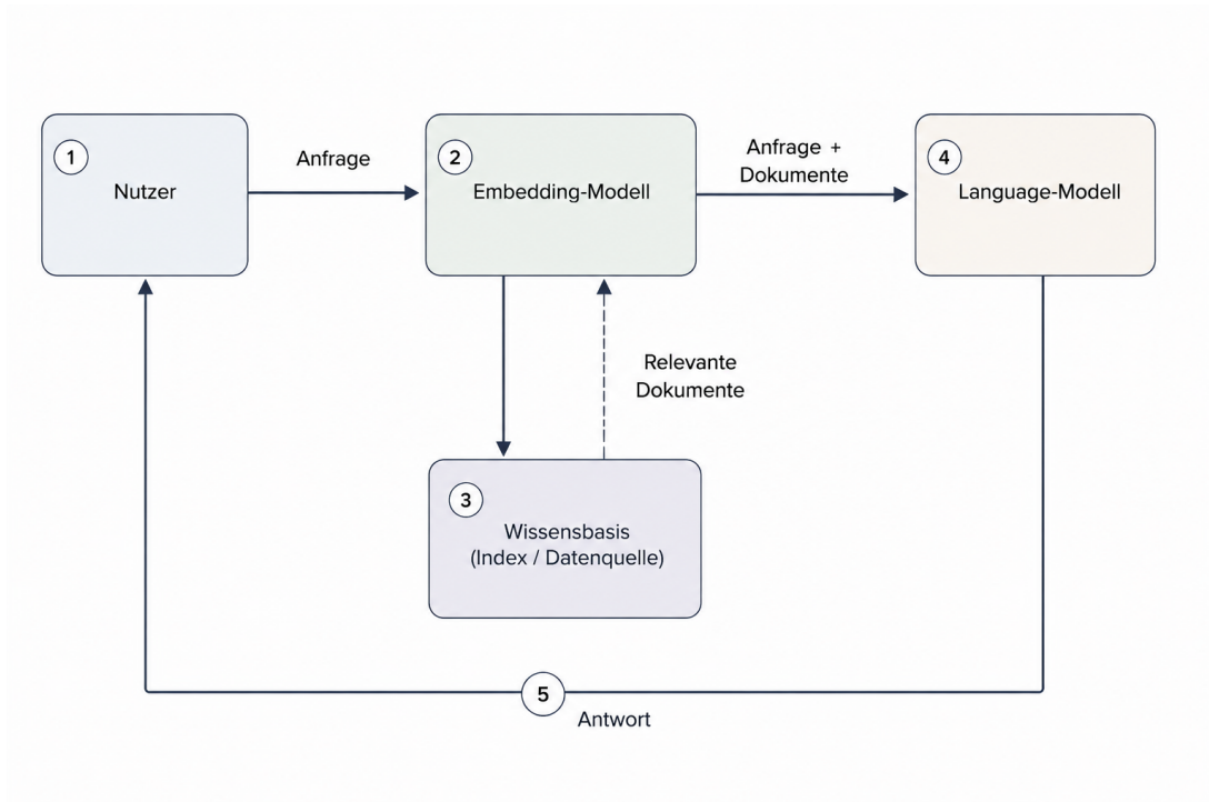
Abbildung 5: Schrittweise Darstellung von Retrieval-Augmented Generation.
