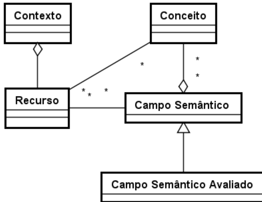
Figura 31.8: Campos semânticos e recursos em UML.
