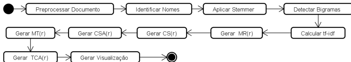
Figura 31.9: Uma instância de um processo de geração de nuvens de rótulo. Adaptado de: F. F. Morgado (2010).
