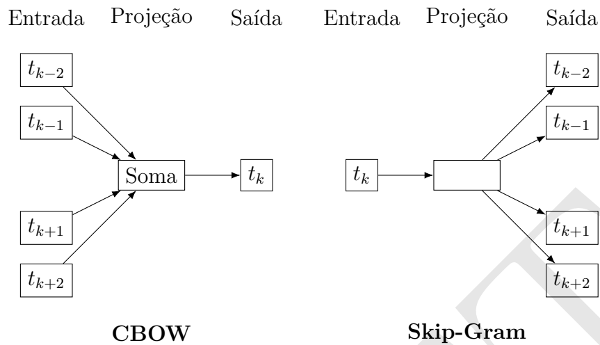
Figura 27.1: Representação dos modos CBOW e Skip-Gram. Fonte: (Bengio et al., 2003)
