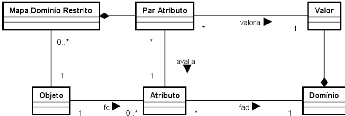
Figura 32.7: Modelo UML que descreve como são construídos os atributos de um objeto
