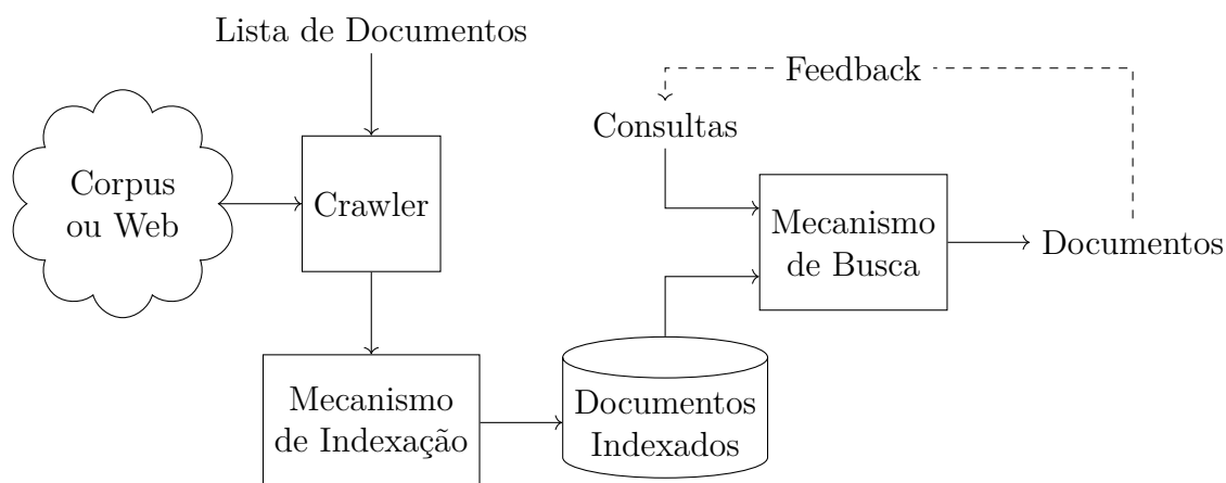
Figura 8.6: Um modelo simples para um sistema de busca.
