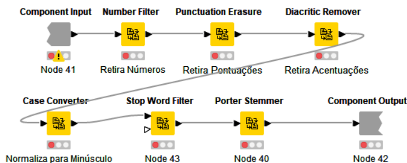
Figura 5.6: Cadeia de pré-processamento em KNIME
