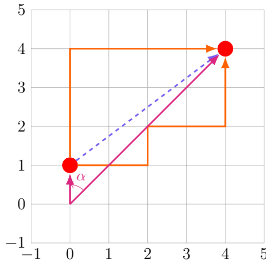
Figura 7.1: Formas de medir a distância entre dois pontos em um espaço. Em magenta a distância do cosseno, em azul tracejado a distância euclidiana e em laranja duas medidas (que vão resultar no mesmo valor) da distância de Manhattan
