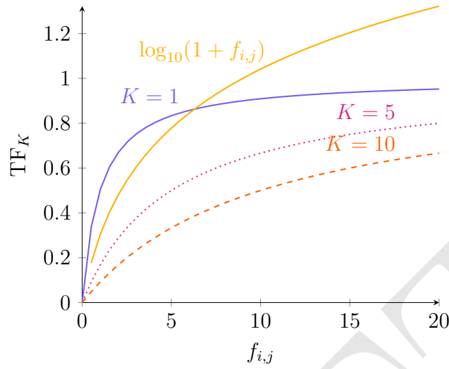
Figura 14.4: Comparação das curvas para \log_{10} e variações de K para TF_K .
