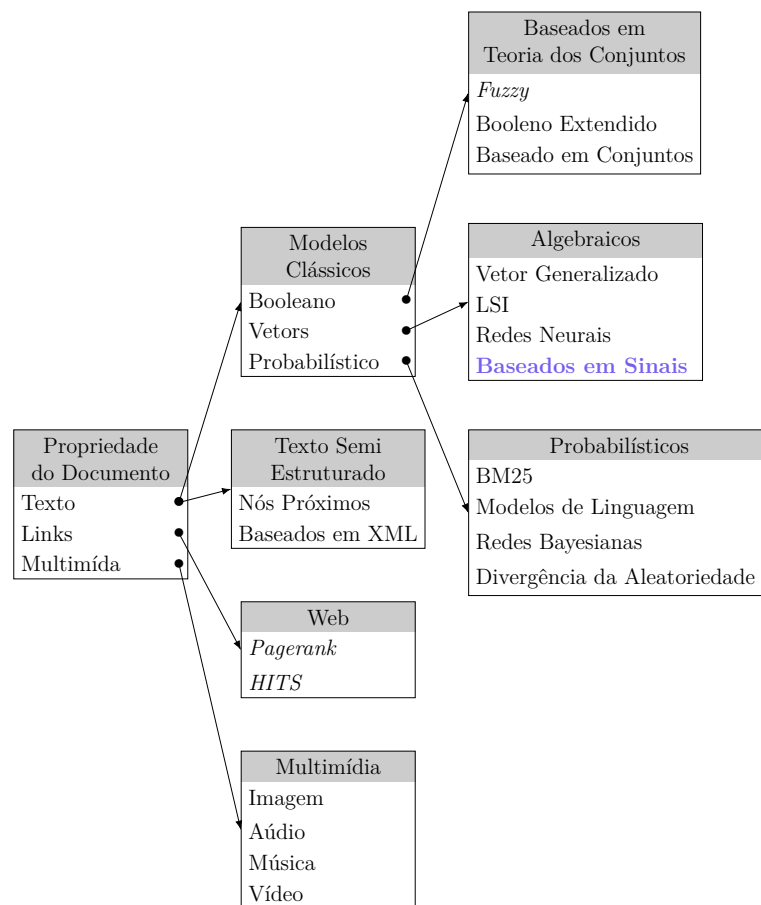
Figura 8.7: Taxonomia da Recuperação da Informação. Fonte: (Baeza-Yates e Ribeiro-Neto, 2011).
