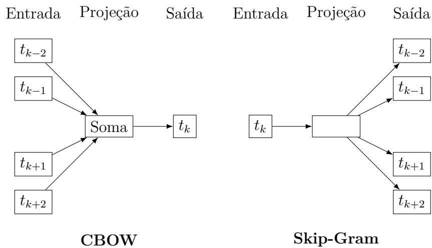
Figura 15.8: Representação dos modos CBOW e Skip-Gram. Fonte: (Bengio et al., 2003)
