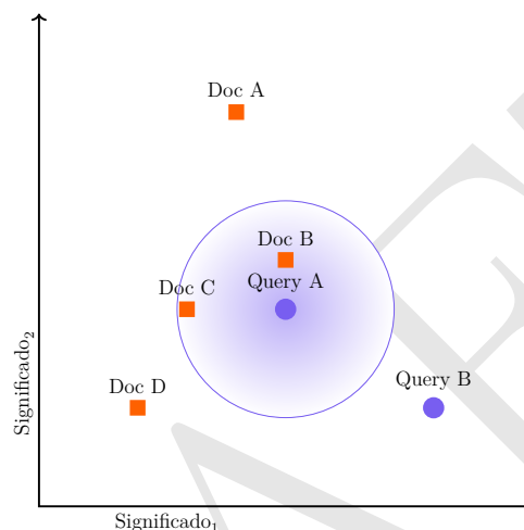
Figura 14.1: A ideia básica do Modelo Vetorial é que os termos do documento, e da consulta, indicam seu significado, e que a similaridade entre a consulta e os documentos da coleção pode ser calculada em um espaço vetorial.
