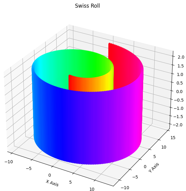
Figura 15.1: O Rolo Suíço é um exemplo clássico usado para ilustrar desafios em técnicas de embedding e redução de dimensionalidade. Ele representa uma superfície bidimensional que foi enrolada em uma terceira dimensão de maneira que não pode ser desdobrada em um plano sem distorção. O objetivo de usar o Rolo Suíço em técnicas de embedding é demonstrar a capacidade de um algoritmo de desenrolar superfícies curvas enquanto preserva a estrutura local dos dados. Fonte: elaboração do autor, baseada em (J. A. Lee e Verleysen, 2007)
