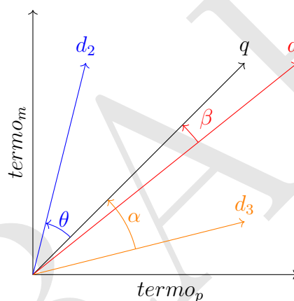
Figura 14.3: Usando o cosseno dos vetores.
