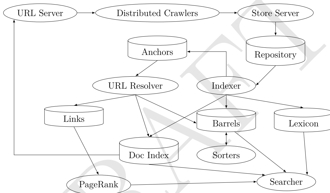
Figura 20.2: Arquitetura original do Google (redesenho). Fonte: (Brin e Page, 1998)
