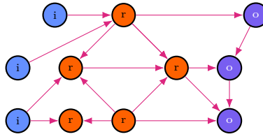
Figura 18.4: Ilustração do primeiro passo do algoritmo HITS, aa construção do base set . No início um mecanismo de busca retorna os nós marcados com r , em laranja, o root set . O conjunto é então estendido com todos os nós apontados por eles, marcados com o , em roxo, e por no máximo k nós que apontam para eles, i , em azul.
