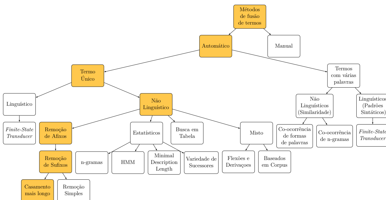
Figura 5.1: Classificação algoritmos de fusão, a partir de Frakes e Baeza-Yates (1992), Galvez, MoyaAnegón e Solana (2005) e Amri e Zenkour (2018). O caminho em amarelo indica os algoritmos de Porter e o RSLP.
