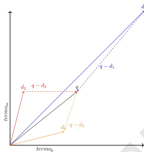
Figura 14.2: Exemplo de problema com o uso do tamanho dos vetores
