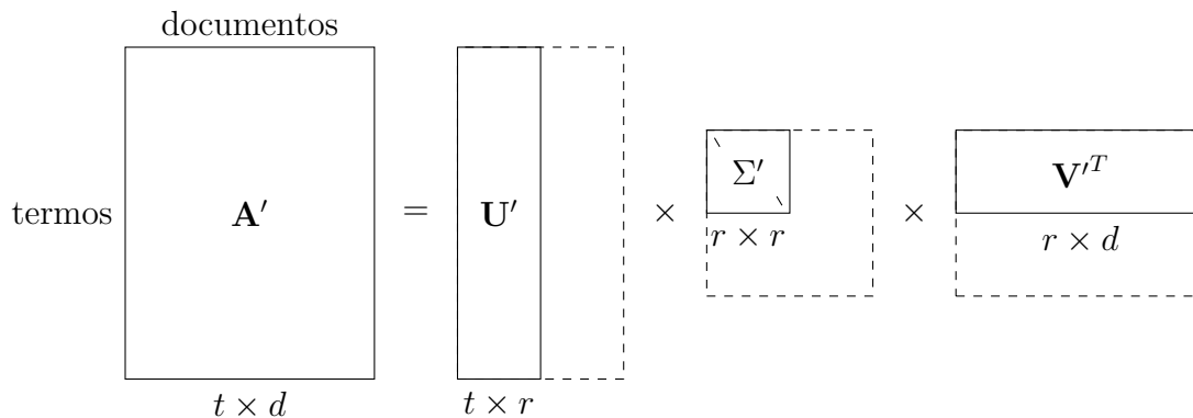
Figura 15.5: Esquema do SVD após a redução de rank . Fonte: (Cohen, 2022)
