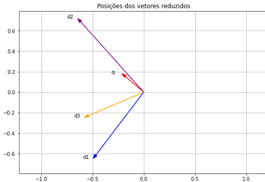
Figura 15.7: Vetores reduzidos do exemplo.
