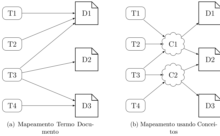
Figura 15.3: Visão abstrata do LSI.
