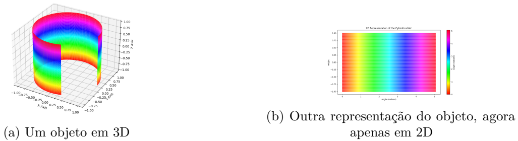
Figura 15.2: Exemplificando o uso de uma transformação de um objeto representado em um espaço tridimensional para um espaço bidimensional.
