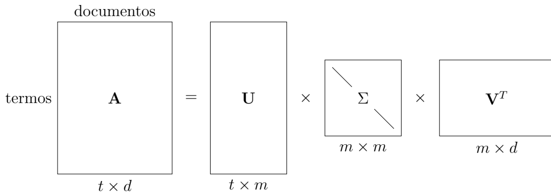
Figura 15.4: Esquema do SVD. Fonte: (Cohen, 2022)
