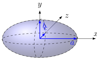
Figura 15.6: Representação de um elipsóide em 3 dimensões mostrando a diferença de tamanho do objeto entre os eixos.
