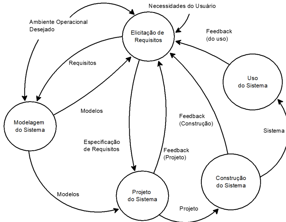
Figura 11.5.: O papel dos requisitos no desenvolvimento do sistema. Fonte:(J. Robertson e S. Robertson, 2006)
