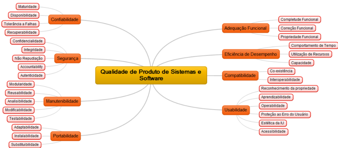
Figura 6.5.: Modelo de Qualidade de Produto de Software da norma ISO 25010. Fonte:(ISO, 2011)
