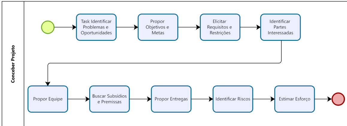
Figura 7.7.: Descrição do sub-processo Conceber Projeto, do processo de criação do Software Project Canvas. Fonte: imagem do autor
