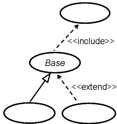
Figura 12.14.: Representações das associações entre casos de uso.
