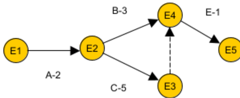
Figura 15.4.: Modelo PERT original para a Tabela 15.1
