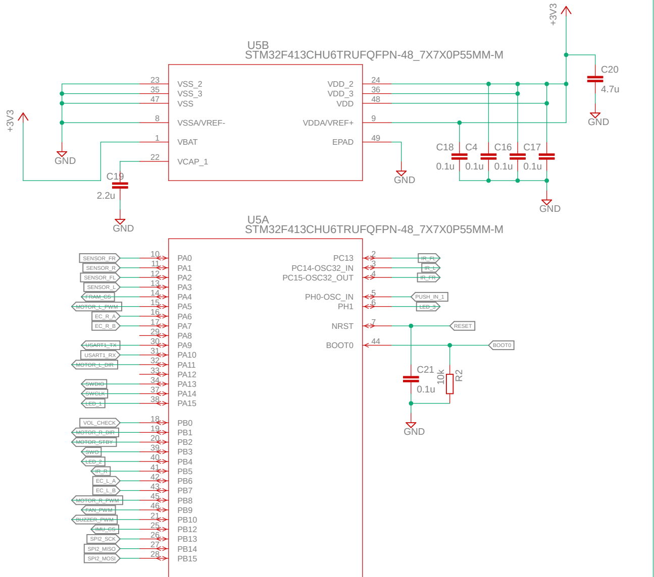
MCU
