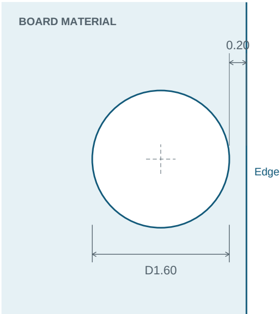
Upper holes - edge detail
