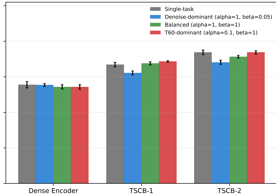
multistats-pooled probe
