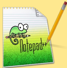
Notepad++
