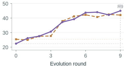
AppWorld · TGC
