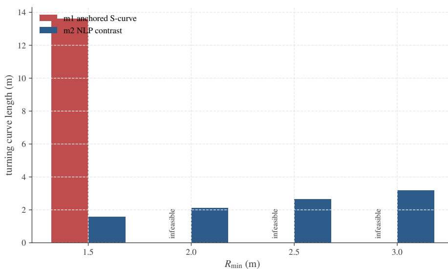
图 13: 问题 4 调头曲线长度在不同转弯半径下界 R_{\min} 下的方法对照。红色为非退化 S 形主调头曲线 (几何半径固定 R_2 = 1.50 m), 蓝色为辅助非线性规划对照; R_{\min} \geq 2.0 m 时超过主曲线几何半径, 说明该外生下界不宜作为主曲线硬约束, 而辅助解始终贴住 R_{\min} 并呈中心塌缩特征。问题 4 可执行性由全队实体无碰撞核验锚定, 不由 R_{\min} 主导。
