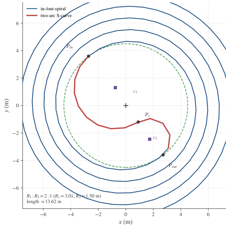
图 9: 问题 4 的 S 形调头曲线几何构造（盘入螺距 1.7\text{ m} ）。蓝色为盘入 / 盘出螺线（关于中心 O 对称），红色为两段相切圆弧组成的调头曲线，前段半径 R_1 = 3.01\text{ m} 为后段 R_2 = 1.50\text{ m} 的两倍 ( 2:1 )，在 P_{\text{in}} 、 P_{\text{out}} 与螺线相切、在内部相切点 P_c ( \|P_c\| = 1.50\text{ m} ) 两弧相切；曲线先内收至 P_c 再外展，全程位于 r = 4.5\text{ m} 调头圆（绿色虚线）内，总长 13.62\text{ m} 。整链经全队实体无碰撞核验通过。
