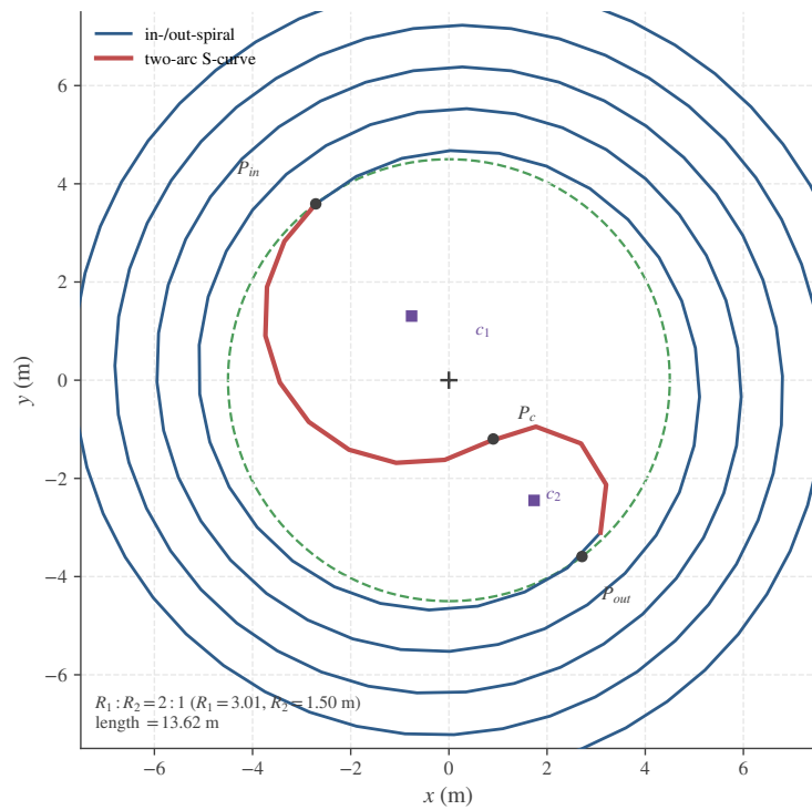
图 9: 问题 4 的 S 形调头曲线几何构造（盘入螺距 1.7 m）。蓝色为盘入 / 盘出螺线（关于中心 O 对称），红色为两段相切圆弧组成的调头曲线，前段半径 R_1 = 3.01 \text{ m} 为后段 R_2 = 1.50 \text{ m} 的两倍 (2:1)，在 P_{in} 、 P_{out} 与螺线相切、在内部相切点 P_c ( \|P_c\| = 1.50 \text{ m} ) 两弧相切；曲线先内收至 P_c 再外展，全程位于 r = 4.5 \text{ m} 调头圆（绿色虚线）内，总长 13.62 m。此为约束系统的非退化分支，整链经全队实体无碰撞核验通过。
