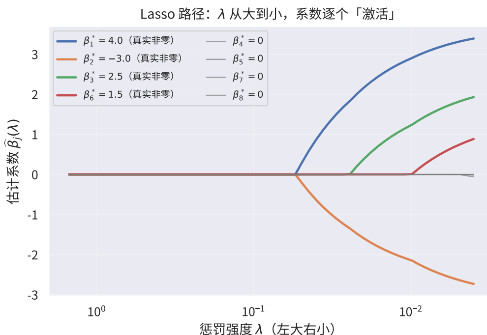
图 8: Lasso 正则化路径（模拟数据，真实系数 4, -3, 2.5, 0, 0, 1.5, 0, 0）： \lambda 从大到小（横轴左大右小），四个真实非零系数（彩线）依次从 0 被「激活」，真实为零的系数（灰线）始终被压在 0 附近——稀疏性不是假设出来的，是 \ell_1 惩罚的几何（菱形约束角）自动选择的。
