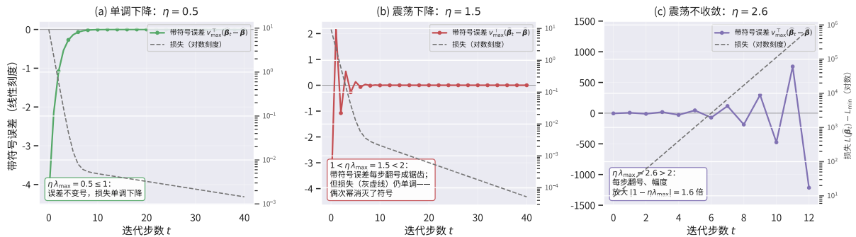
图 5: 带符号误差 (彩色实线, 左轴, 线性刻度) 与损失 (灰虚线, 右轴, 对数刻度) 随迭代步数 t 的三档形态 (同一二次问题、同一初值、仅改变 \eta ): (a) 单调下降—— \eta\lambda_{\max} \leq 1 , 最大特征方向误差不变号, 损失单调; (b) 震荡下降—— 1 < \eta\lambda_{\max} < 2 , 带符号误差每步翻号成锯齿, 但损失因偶次幂仍单调下滑; (c) 震荡不收敛—— \eta\lambda_{\max} > 2 , 误差每步翻号、幅度以 |1 - \eta\lambda_{\max}| 倍放大, 损失爆炸。
