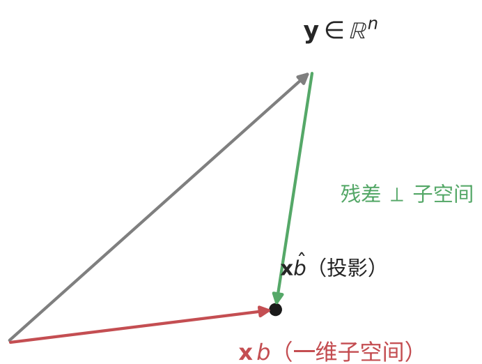
(c) 几何：最小二乘 = 正交投影
