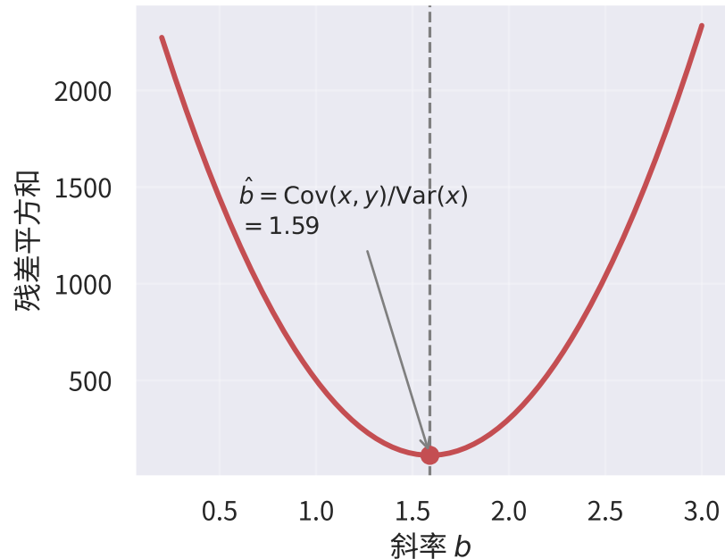
(b) 目标函数：单峰、可解
