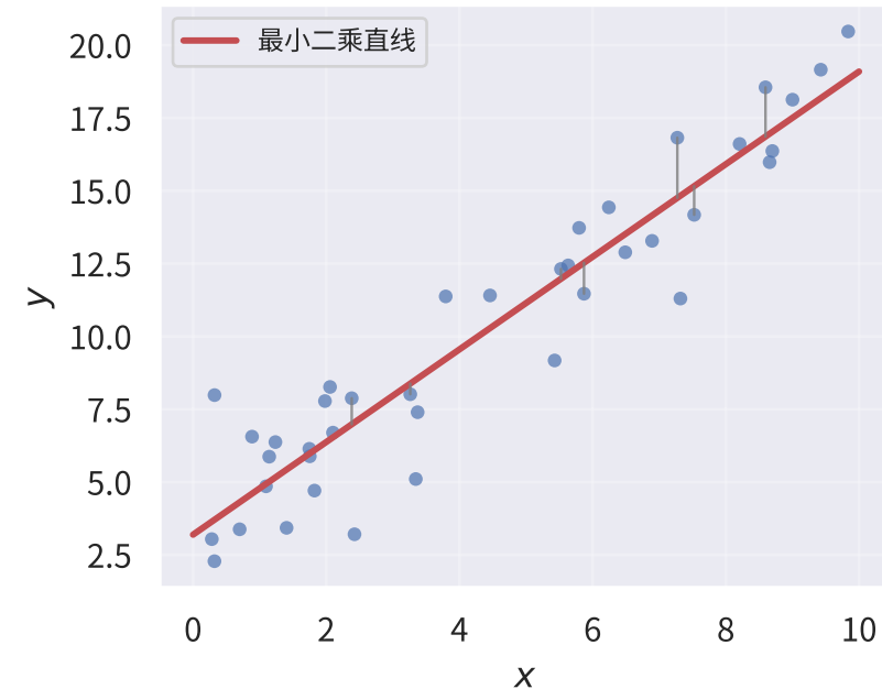
(a) 拟合：残差平方和最小
