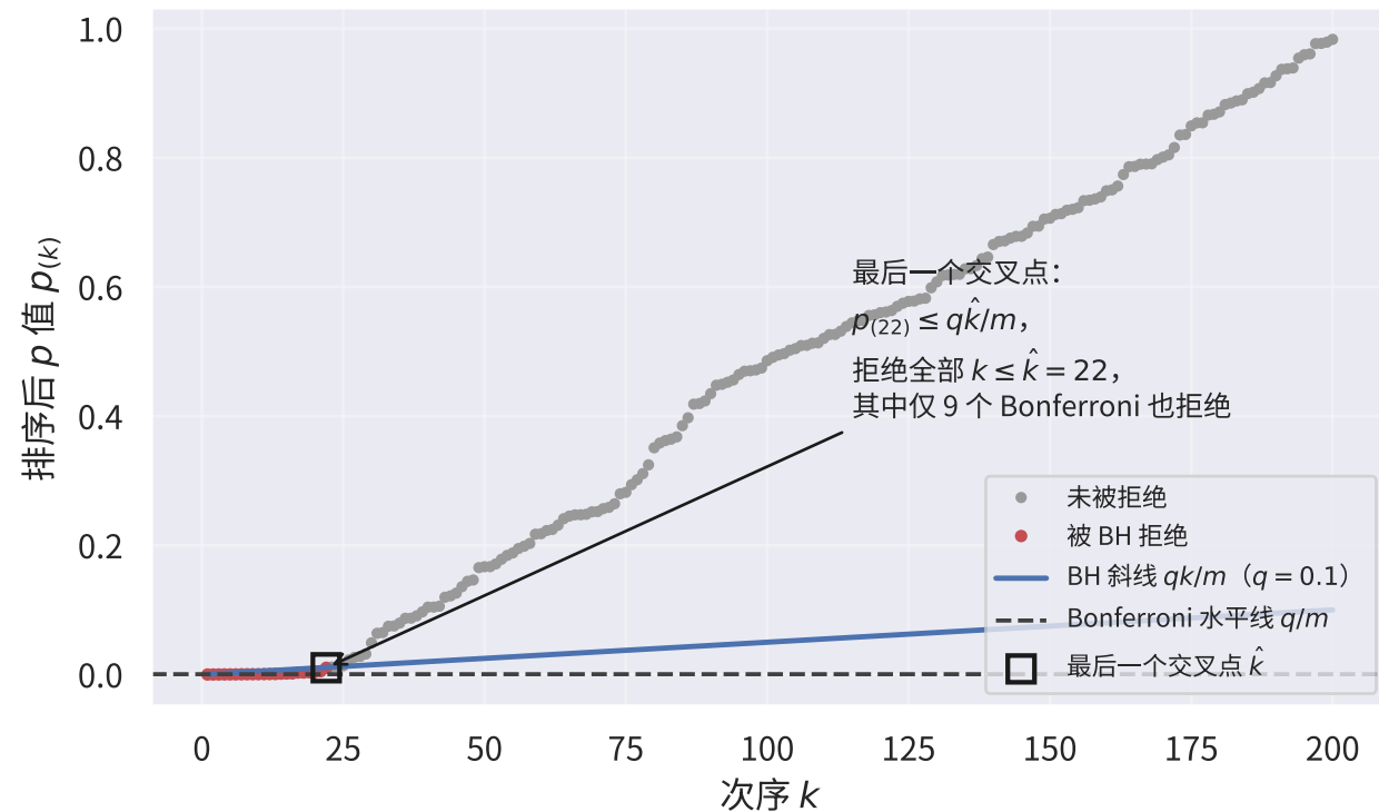
(a) BH 的几何：斜线放松阈值，Bonferroni 是水平线
