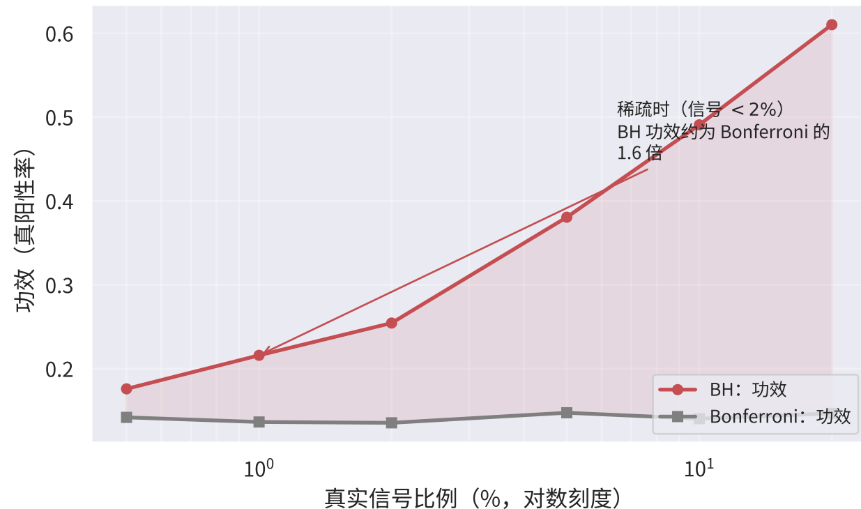
(b) 功效对比 ( m = 1000 , q = 0.05 , 200 次重复； 两种方法的 FDR 均不超过 q )
