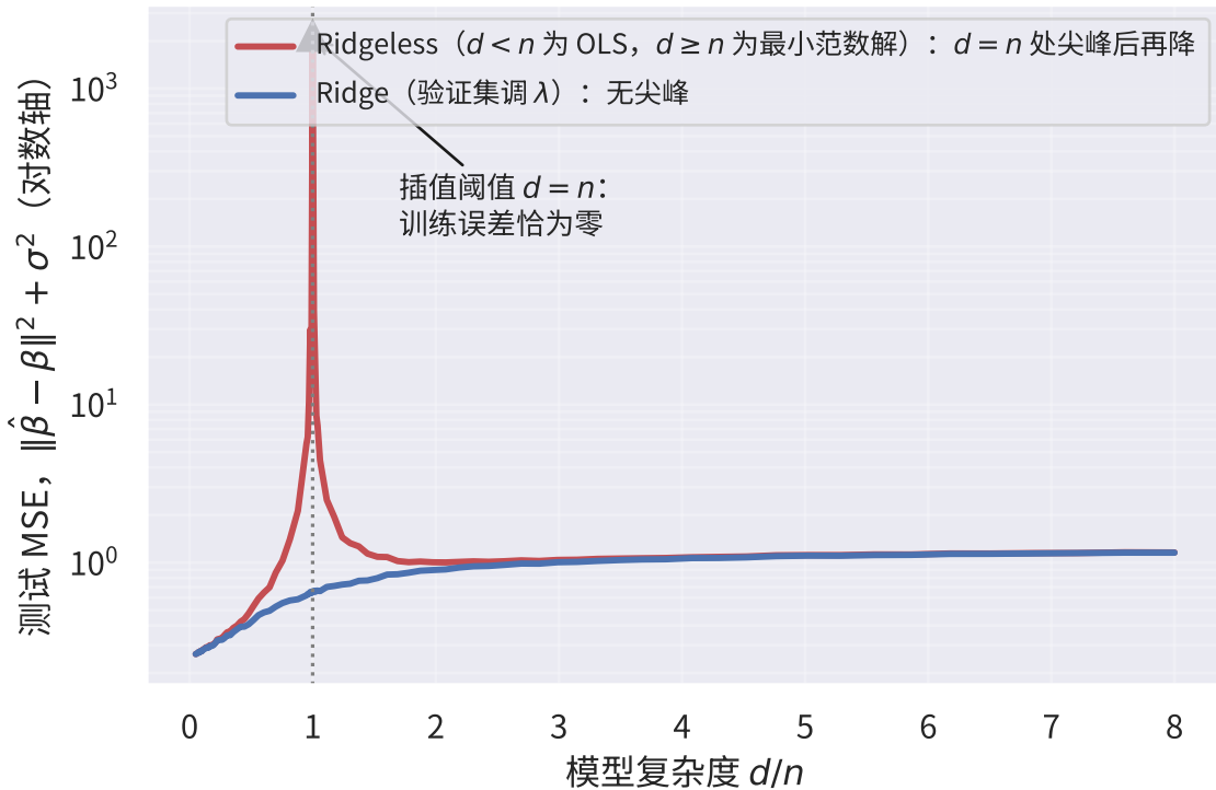
Double descent 模拟复现 ( n = 200 , 每个 d 取 25 次设计抽样)
