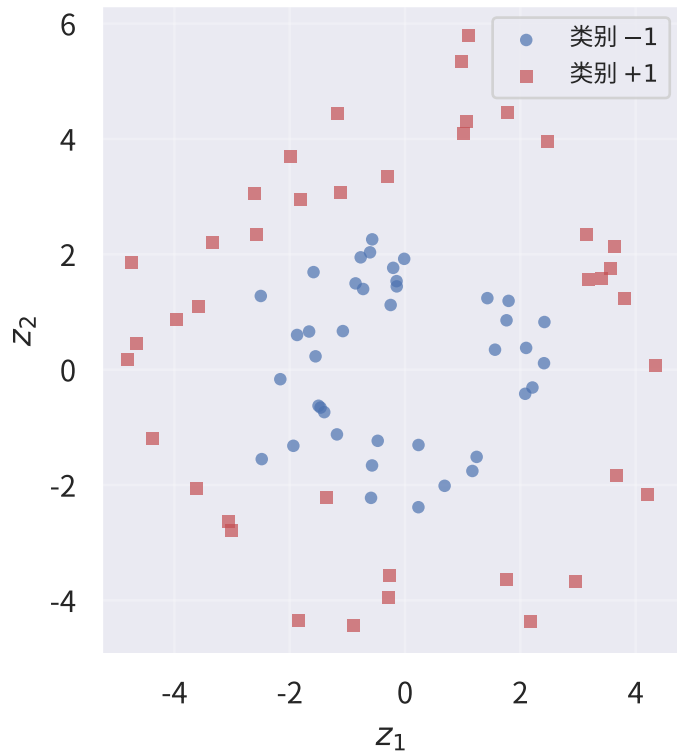
(a) 原始空间 z : 线性不可分
