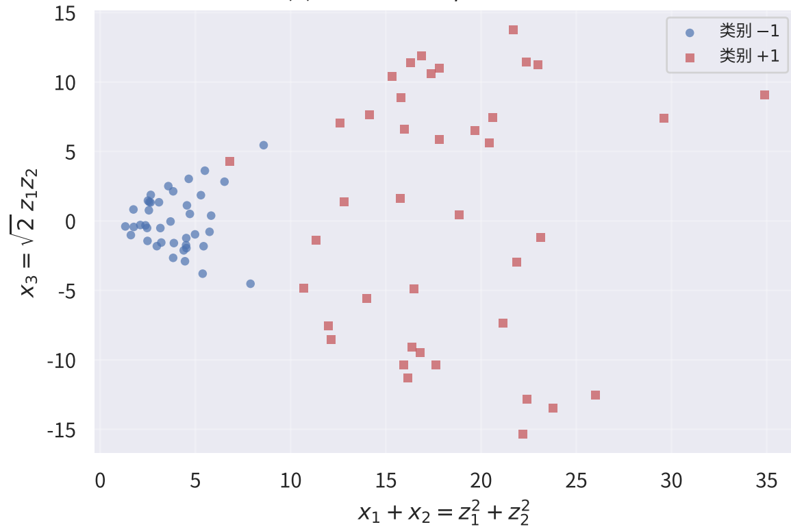
(b) 特征空间 x = \phi(z) : 线性可分
