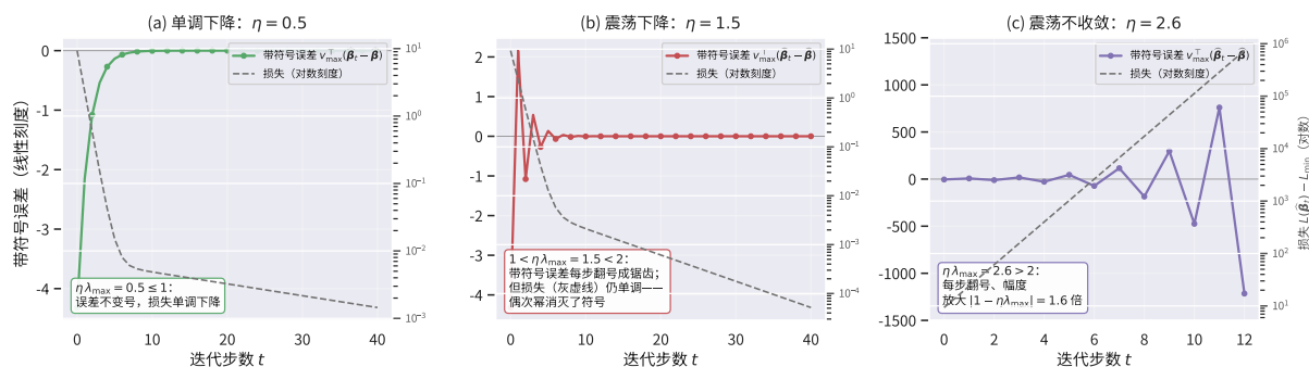
图 5：带符号误差（彩色实线，左轴，线性刻度）与损失（灰虚线，右轴，对数刻度）随迭代步数 t 的三档形态（同一二次问题、同一初值、仅改变 \eta ）：(a) 单调下降—— \eta\lambda_{\max} \leq 1 ，最大特征方向误差不变号，损失单调；(b) 震荡下降—— 1 < \eta\lambda_{\max} < 2 ，带符号误差每步翻号成锯齿，但损失因偶次幂仍单调下滑；(c) 震荡不收敛—— \eta\lambda_{\max} > 2 ，误差每步翻号、幅度以 |1 - \eta\lambda_{\max}| 倍放大，损失爆炸。
