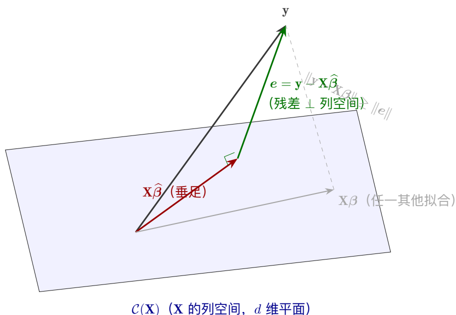
图 4: 最小二乘的几何: \mathbf{y} 到列空间 \mathcal{C}(\mathbf{X}) 的垂足是 \mathbf{X}\hat{\beta} 。垂线段 e 是最短残差 (绿); 任何其他拟合值 \mathbf{X}\beta (灰) 到 \mathbf{y} 的斜线都更长——垂直即最优。
