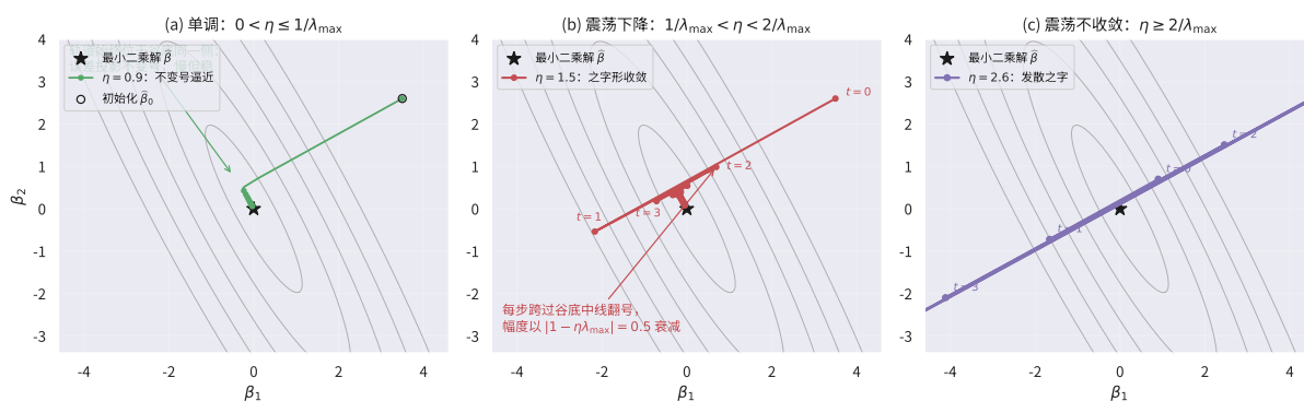
图 6: 梯度下降在二次损失（条件数 \kappa = 25 的椭圆谷）上的三条轨道，与步长三档一一对应：(a) \eta = 0.9 \leq 1/\lambda_{\max} ：轨道不跨谷底中线、不变号逼近，但沿「瘦」方向缓慢爬行；(b) 1/\lambda_{\max} < \eta = 1.5 < 2/\lambda_{\max} ：轨道每步跨过谷底翻号，之字形幅度以 |1 - \eta\lambda_{\max}| = 0.5 衰减——震荡下降；(c) \eta = 2.6 > 2/\lambda_{\max} ：每步翻号、幅度放大 1.6 倍，数步内飞出视野。
