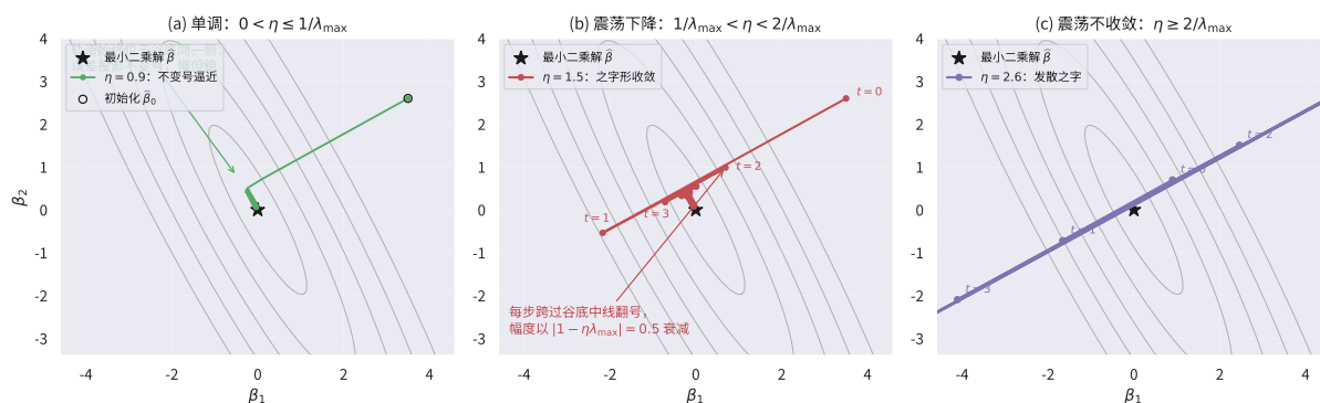
图 6: 梯度下降在二次损失 (条件数 \kappa = 25 的椭圆谷) 上的三条轨道, 与步长三档一一对应: (a) \eta = 0.9 \leq 1/\lambda_{\max} : 轨道不跨谷底中线、不变号逼近, 但沿「瘦」方向缓慢爬行; (b) 1/\lambda_{\max} < \eta = 1.5 < 2/\lambda_{\max} : 轨道每步跨过谷底翻号, 之字形幅度以 |1 - \eta\lambda_{\max}| = 0.5 衰减——震荡下降; (c) \eta = 2.6 > 2/\lambda_{\max} : 每步翻号、幅度放大 1.6 倍, 数步内飞出视野。
