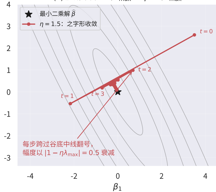
(b) 震荡下降: 1/\lambda_{\max} < \eta < 2/\lambda_{\max}
