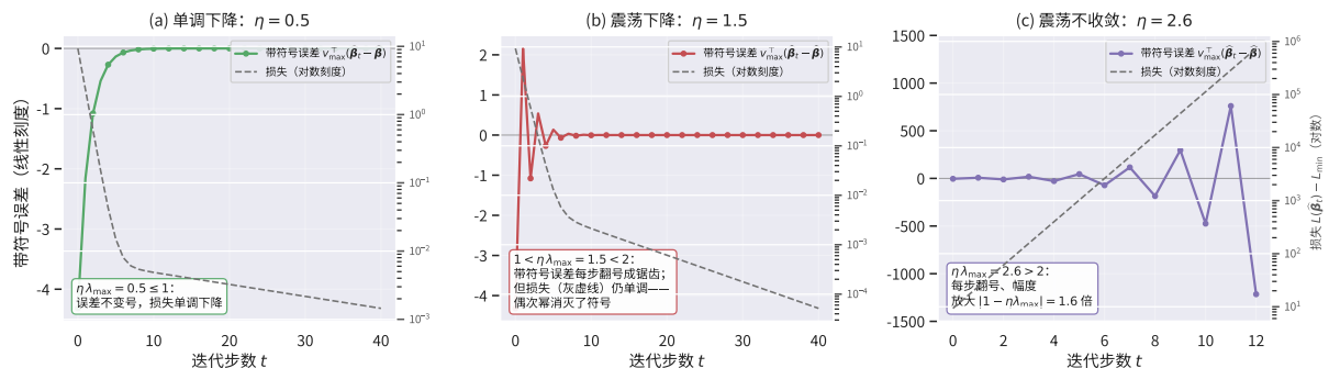
图 5: 带符号误差（彩色实线，左轴，线性刻度）与损失（灰虚线，右轴，对数刻度）随迭代步数 t 的三档形态（同一二次问题、同一初值、仅改变 \eta ）：(a) 单调下降—— \eta\lambda_{\max} \leq 1 ，最大特征方向误差不变号，损失单调；(b) 震荡下降—— 1 < \eta\lambda_{\max} < 2 ，带符号误差每步翻号成锯齿，但损失因偶次幂仍单调下滑；(c) 震荡不收敛—— \eta\lambda_{\max} > 2 ，误差每步翻号、幅度以 |1 - \eta\lambda_{\max}| 倍放大，损失爆炸。
