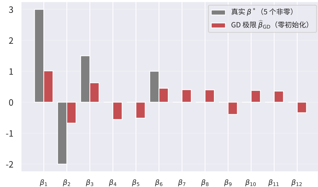
(a) GD 自动找到「能量集中」的插值解
