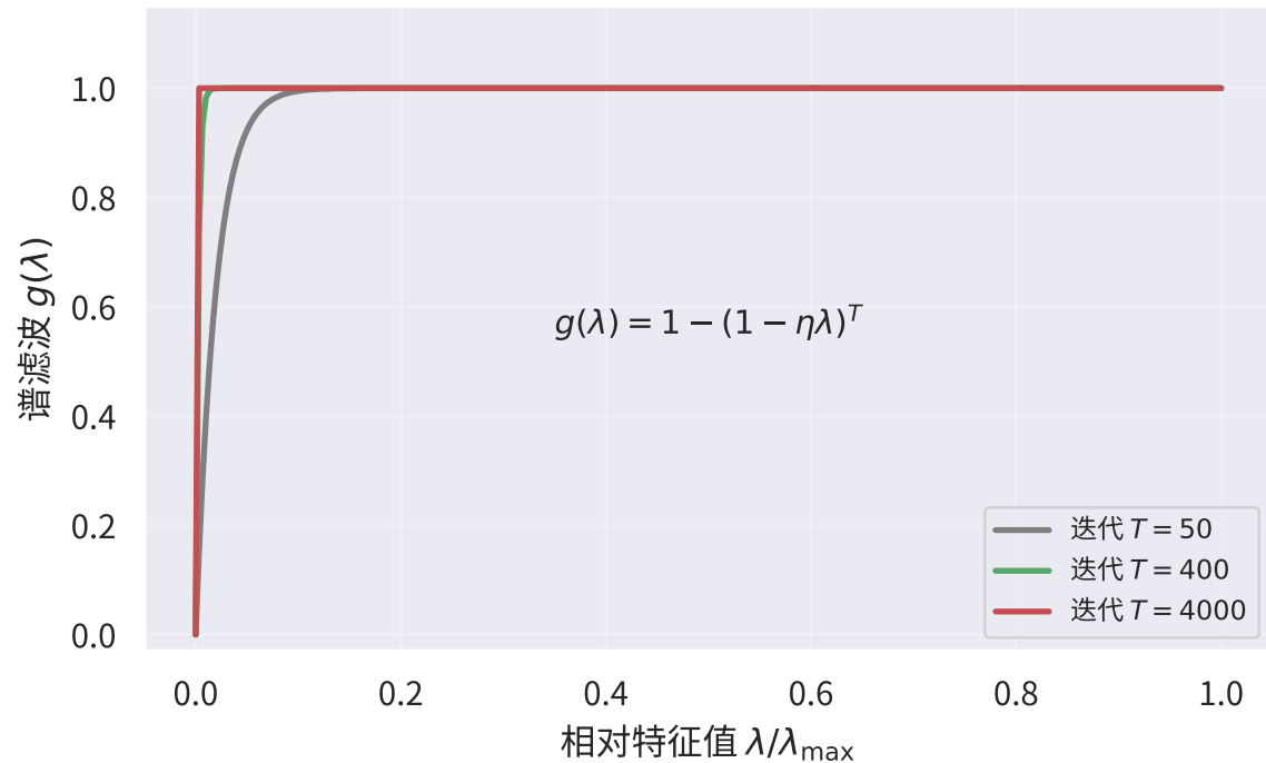
(b) GD 极限 = 谱域「低通滤波器」
