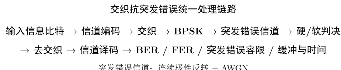
图 9.1: 交织抗突发错误仿真链路
