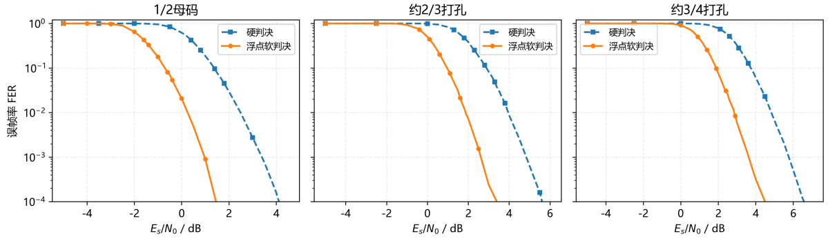
图 5.5: 硬判决与浮点软判决的帧错误率比较
