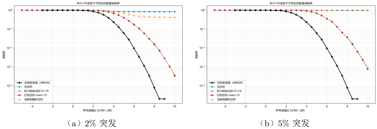
图 9.2: 分块 BCH 在两档突发长度下的误帧率
