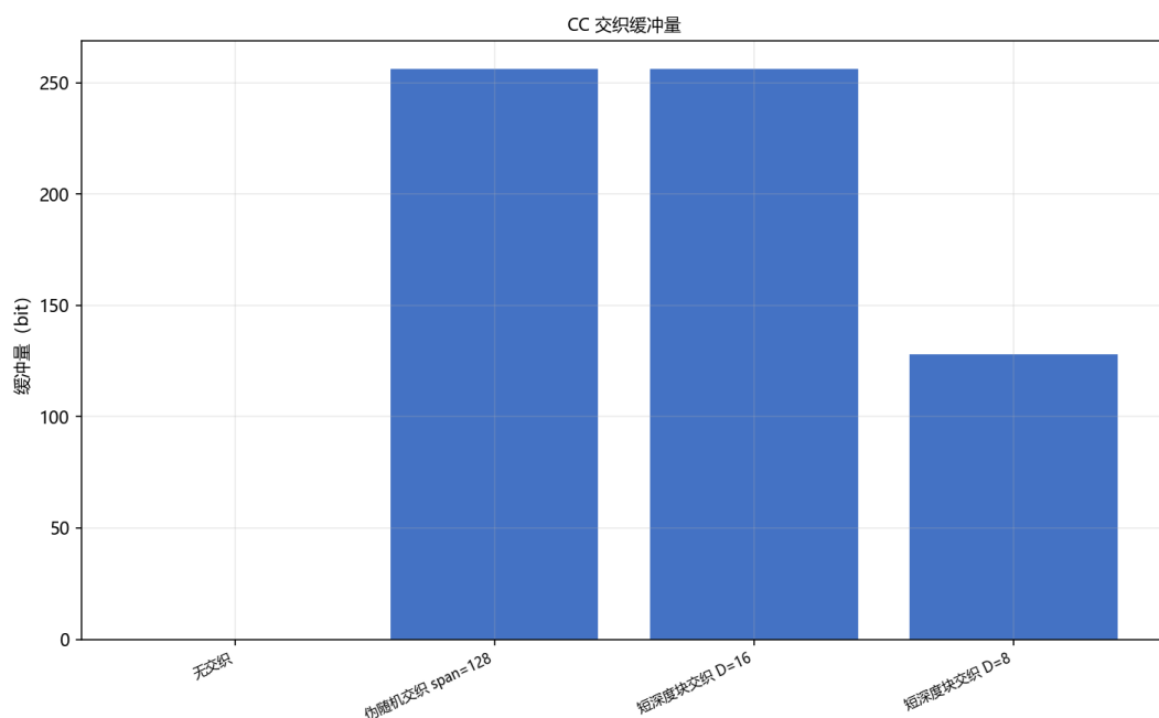
图 9.15: 卷积码交织配置的结构缓存量
