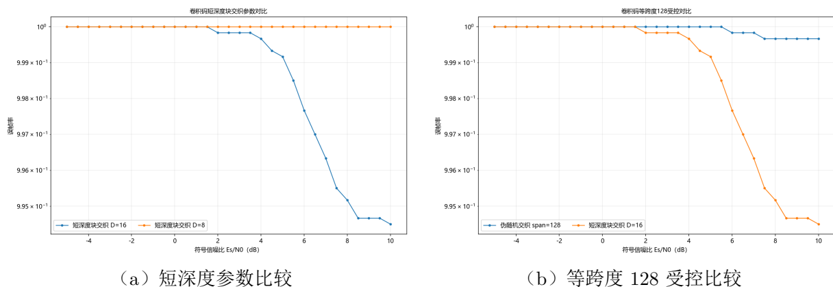
图 9.13: 卷积码短深度与等跨度交织比较
