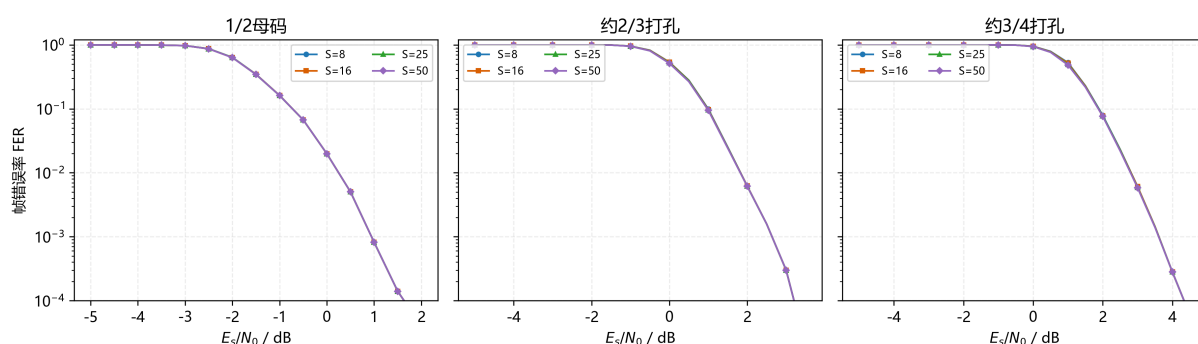
图 5.12: 不同滑动步长对滑窗译码 FER 的影响
