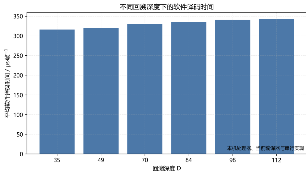
图 5.7: 不同回溯深度下的软件译码时间
