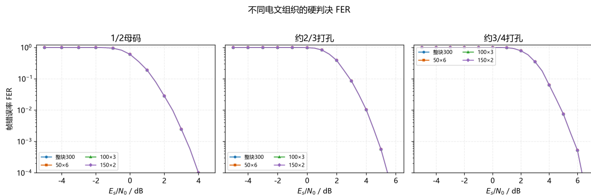
图 5.15: 不同电文组织的硬判决帧错误率
