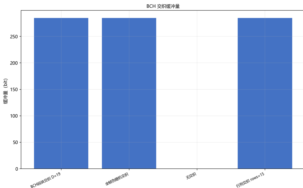
图 9.8: BCH 交织配置的结构缓存量
