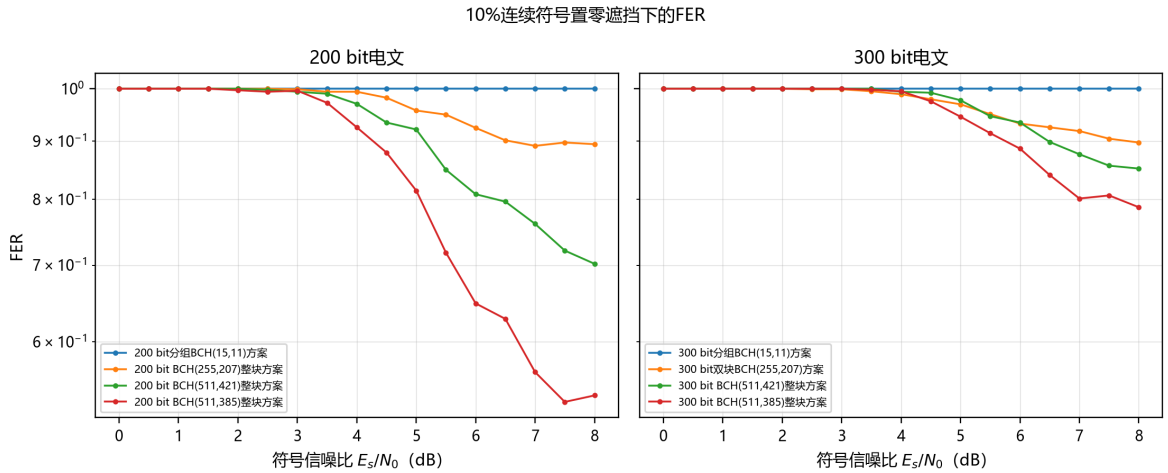
图 4.9: 约 10% 连续符号置零遮挡下的帧错误率
