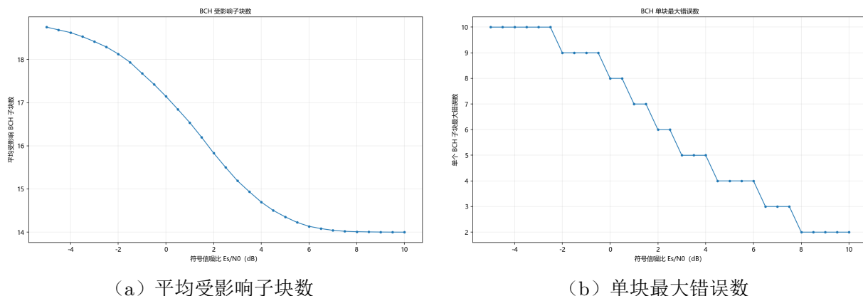
图 9.7: 5% 突发条件下 BCH 错误分散机理证据
