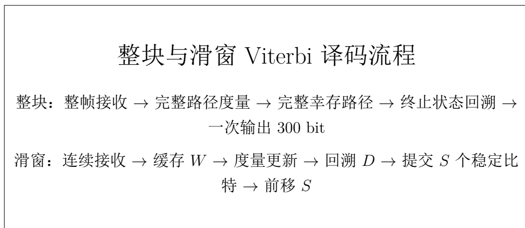
图 5.3: 整块与滑窗 Viterbi 译码流程
