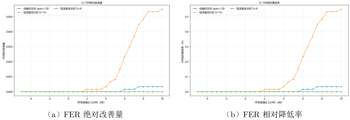
图 9.14: 5% 突发条件下卷积码交织的 FER 改善
