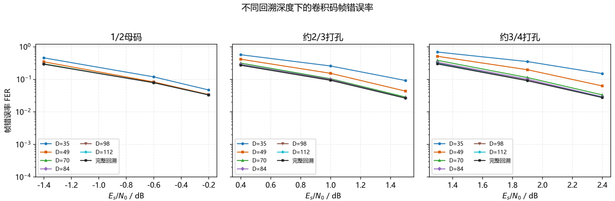
图 5.6: 不同回溯深度下的卷积码帧错误率
