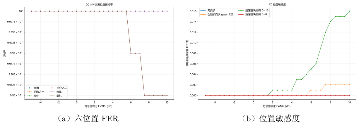
图 9.12: 5% 突发条件下卷积码突发位置敏感性
