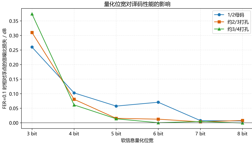
图 5.10: 软信息量化位宽的 FER=0.1 性能损失
