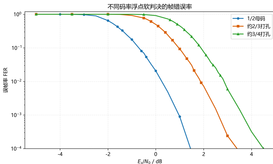
图 5.4: 不同码率浮点软判决的帧错误率
