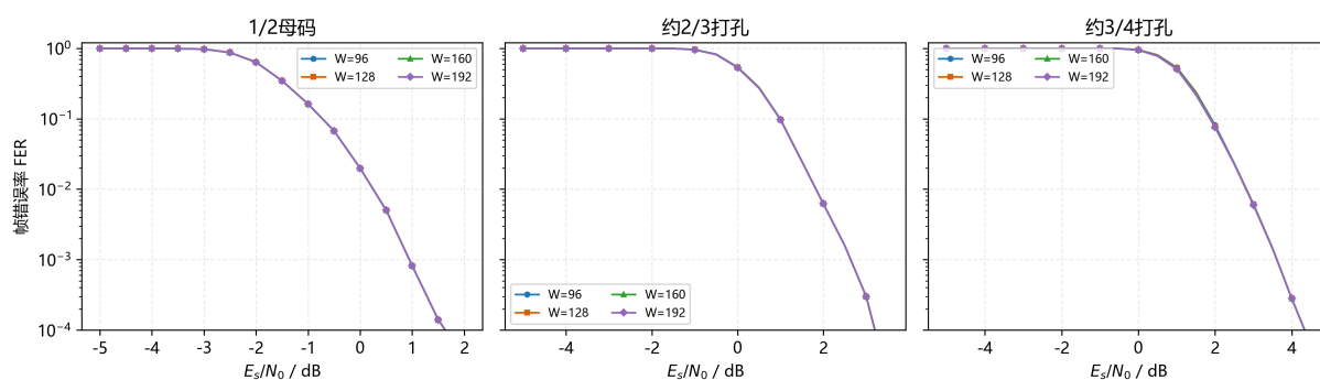
图 5.11: 不同窗口长度对滑窗译码 FER 的影响
