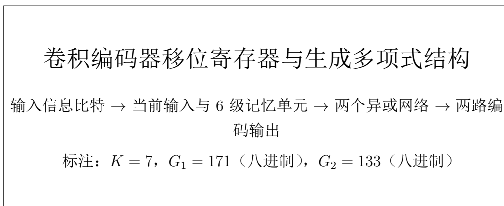
图 5.1: 卷积编码器移位寄存器与生成多项式结构
