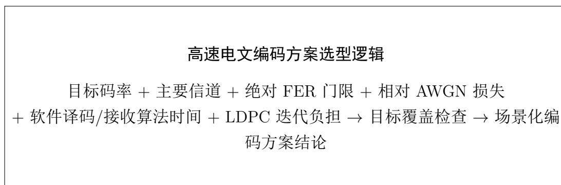
图 7.14: 高速电文多信道编码方案选型逻辑
