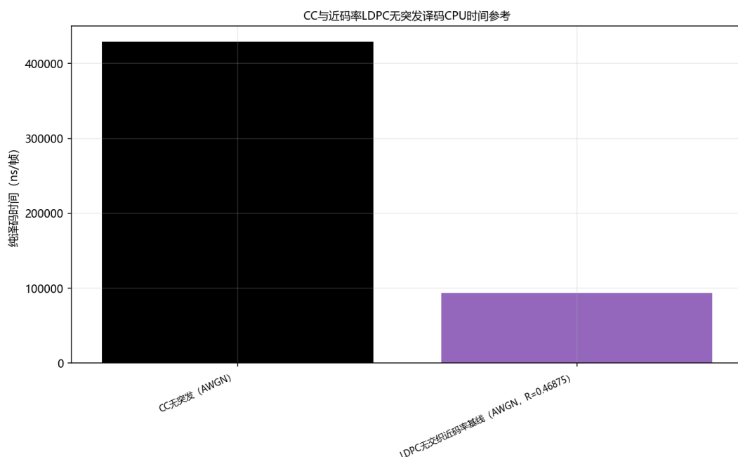
图 9.16: 卷积码与 LDPC 无交织、无突发 AWGN 软件译码 CPU 时间参考
