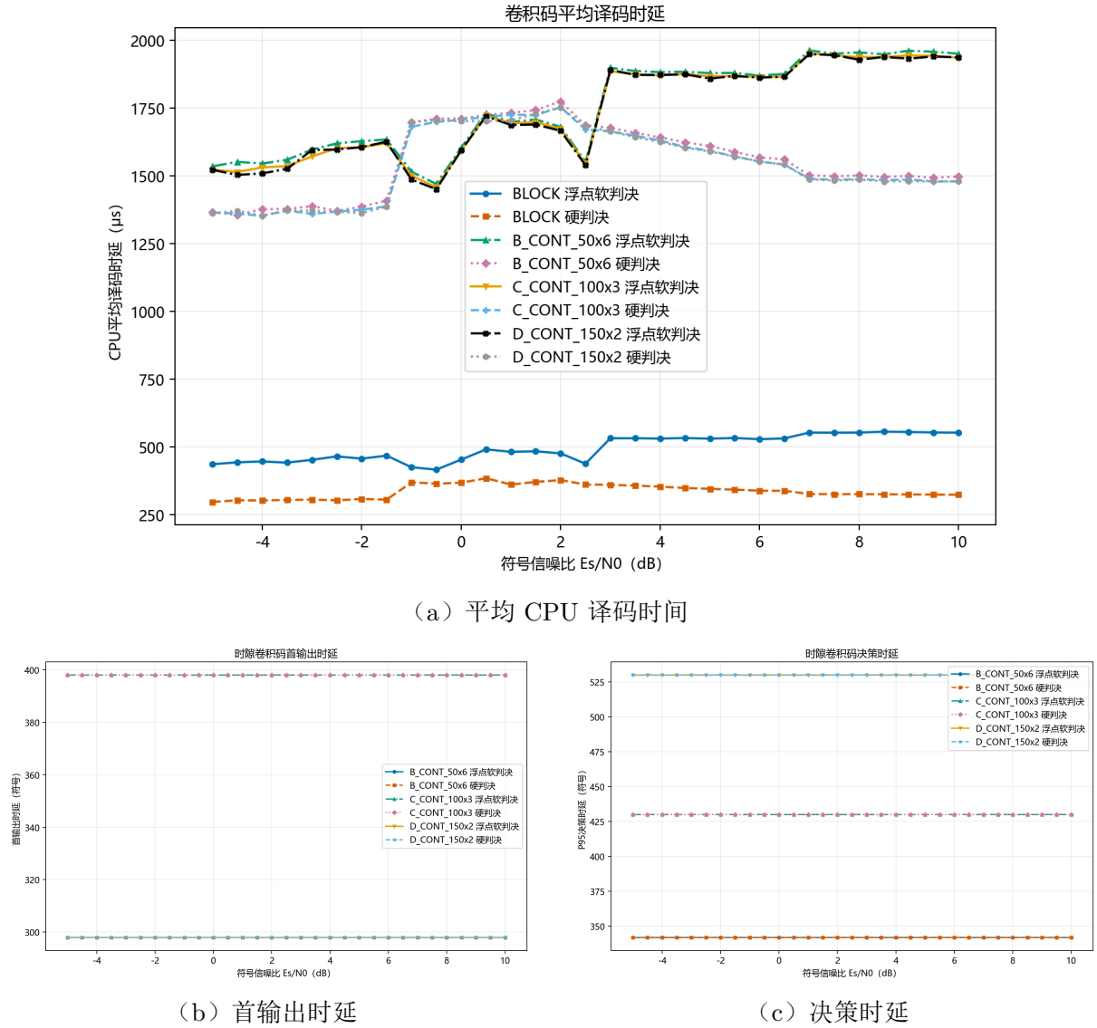
图 8.8: 卷积码 Viterbi 译码的软件时间与流式输出时延
