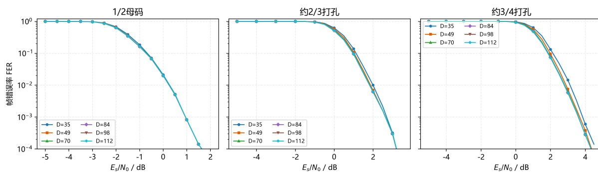
图 5.13: 不同回溯深度对滑窗译码 FER 的影响
