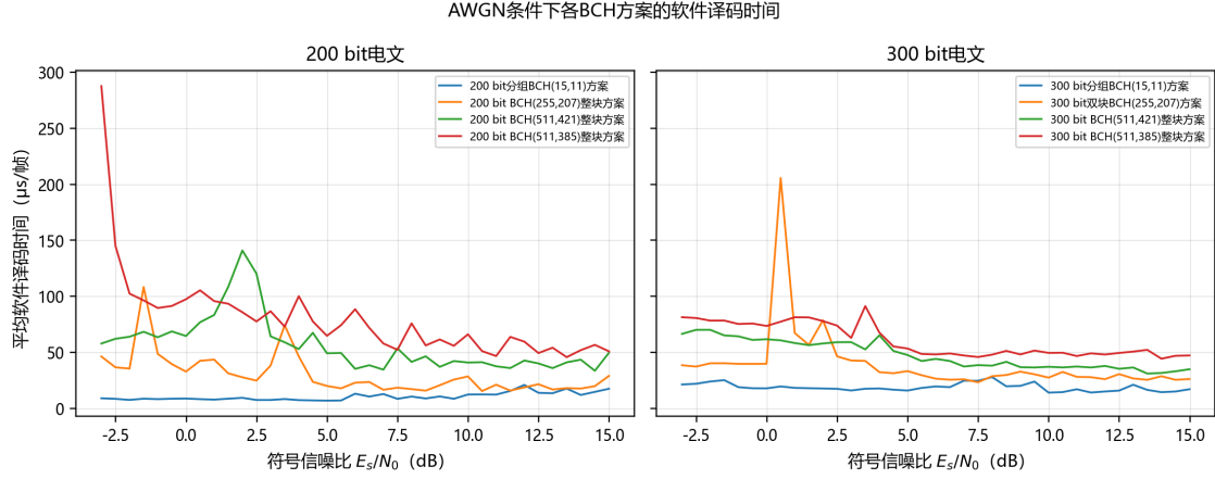
图 4.5: AWGN 条件下各 BCH 方案的软件译码时间
