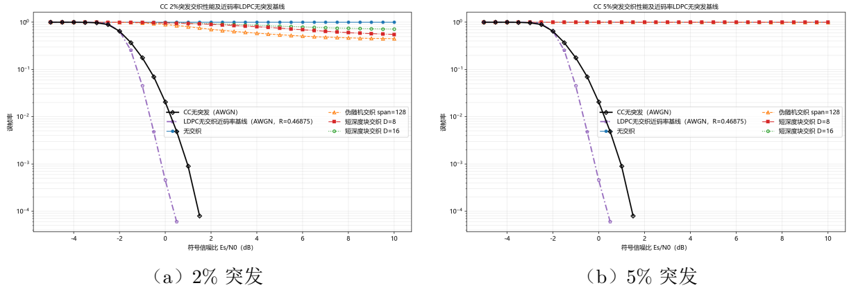
图 9.9: 卷积码在两档突发长度下的误帧率。LDPC 曲线为无突发 AWGN 近码率基线, 不表示 LDPC 经历突发错误
