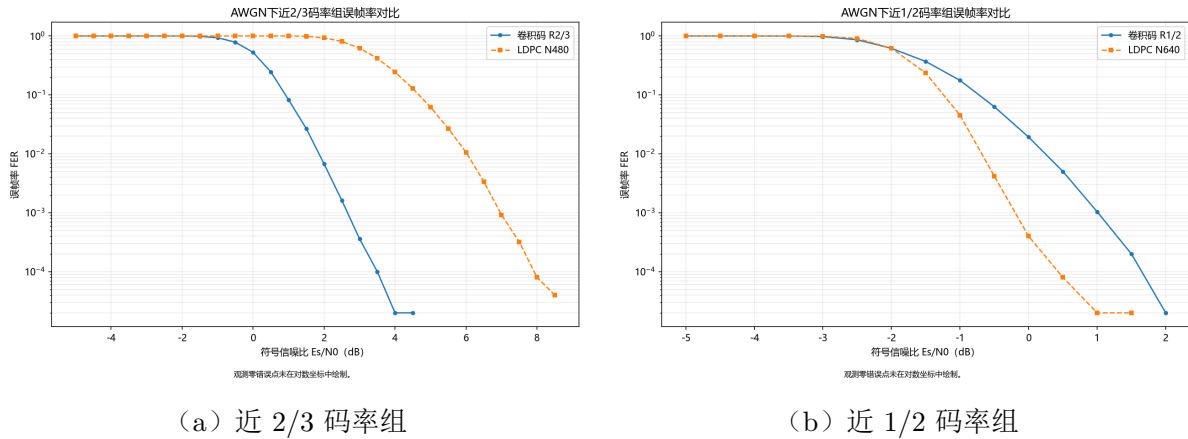
图 7.3: 不同近似码率组在 AWGN 信道下的误帧性能
