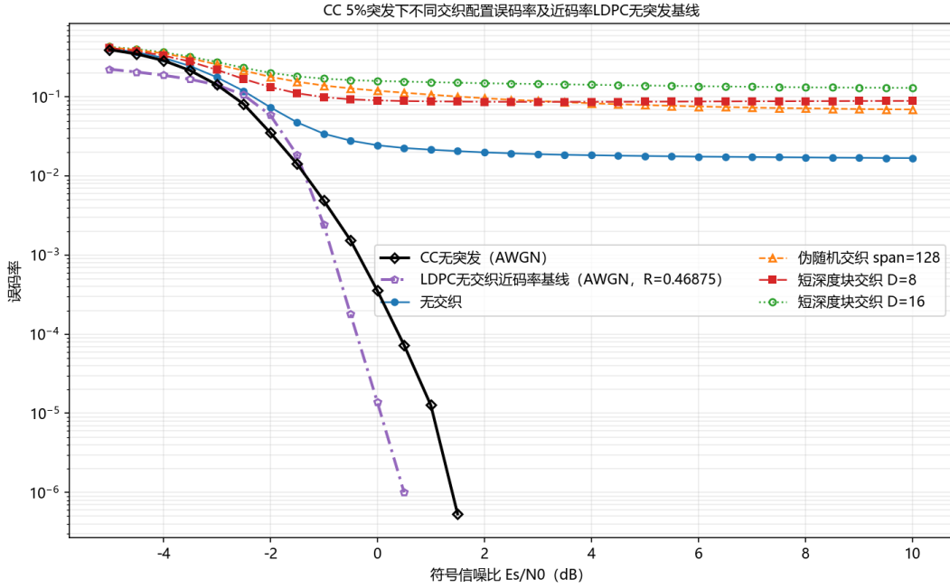
图 9.10: 5% 突发条件下卷积码不同交织配置的误码率。LDPC 曲线为无突发 AWGN 近码率基线
