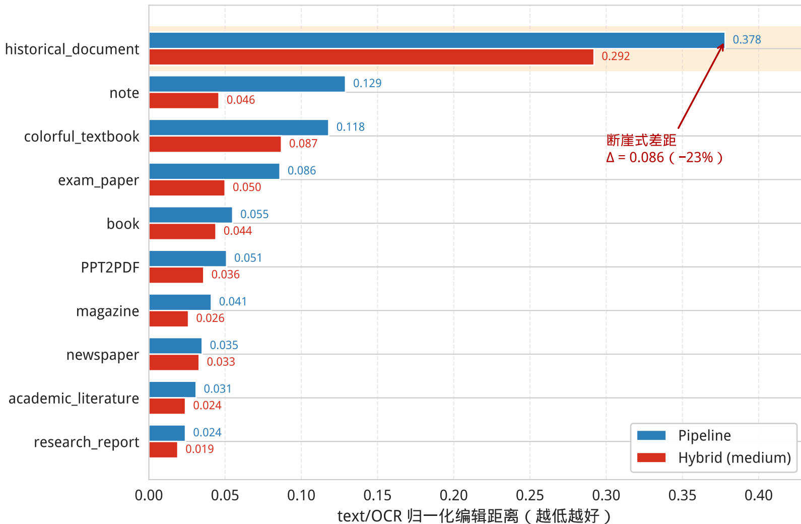
高难度样本断崖式差异：Pipeline vs Hybrid ( 全量 1651 页，按 data_source )
