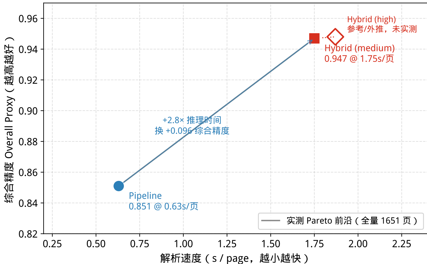
综合精度 vs 解析速度 Trade-off ( OmniDocBench 全量 1651 页 )
