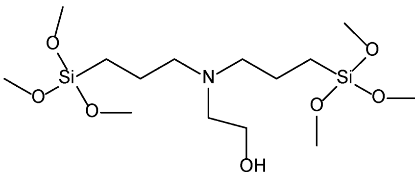
- 2-[Bis[3-(triethoxysilyl)propyl]amino]-ethanol
