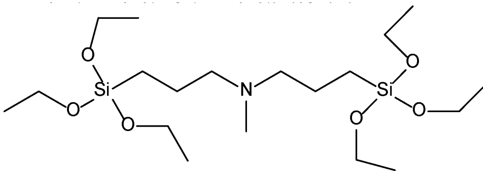
- 2-[Bis[3-(triethoxysilyl)propyl]amino]-ethanol
