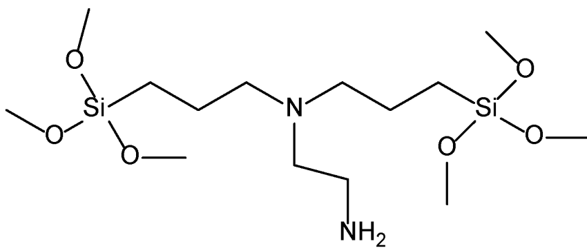
- N1,N1-Bis[3-(triethoxysilyl)propyl]-1,2-ethanediamin,
