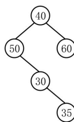
二叉树 T2
