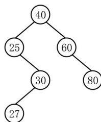
二叉树 T1
