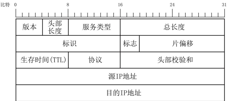
(a) IP 分组头结构
