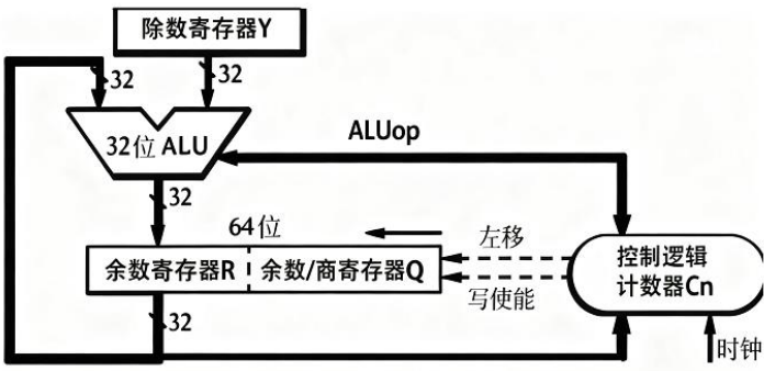
题 44（b）图 补码除法器逻辑结构
