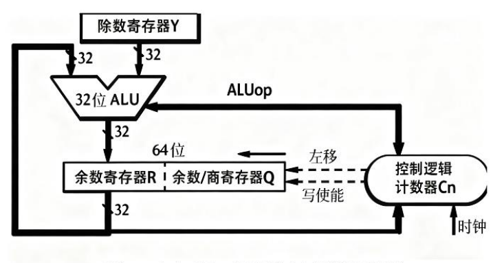
题 44（b）图 补码除法器逻辑结构
