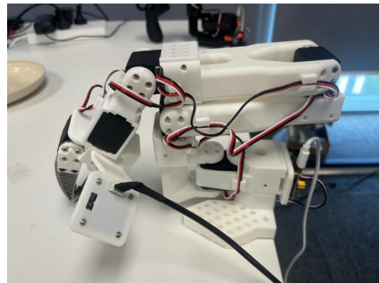
(b) 从动端机械臂
