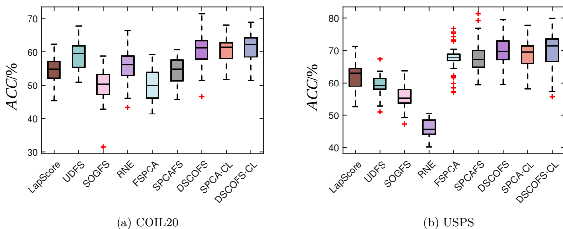
图 6.3 模型稳定性分析结果
