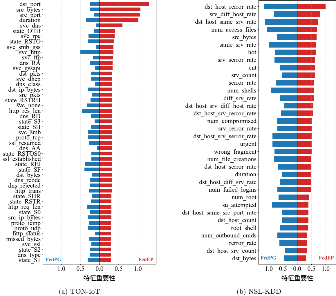
图 3.1 TON-IoT 和 NSL-KDD 数据集的特征重要性可视化结果
