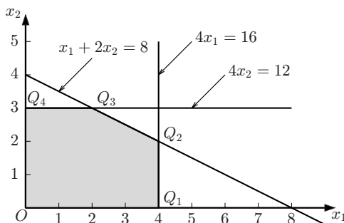
图 1.1 可行域
