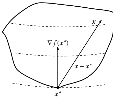
图 3.3 凸函数性质
