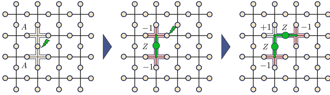
図 4.2: 位相エラーは格子上の Z -鎖として表され、スタビライザーが A_v = -1 となるシンドロームは鎖の端点に現れる。
