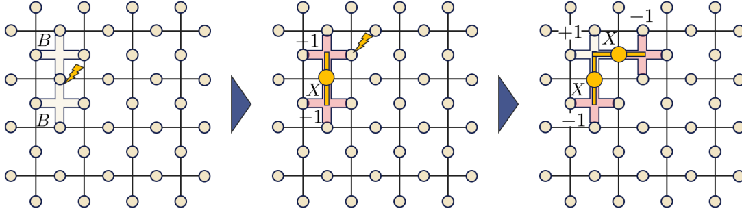
図 4.6: シフトエラーは双対格子上的 X -鎖として表され、そのシンδροームは鎖の端点に対応する面に現れる。
