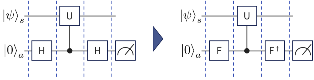
図 2.1: \mathbb{F}_p における Hadamard テストの回路図。 \mathbb{F}_2 ではエルミートな H で表される Hadamard ゲートだったが、 \mathbb{F}_p では非エルミートな F で表される離散フーリエ変換ゲートが用いられる。
