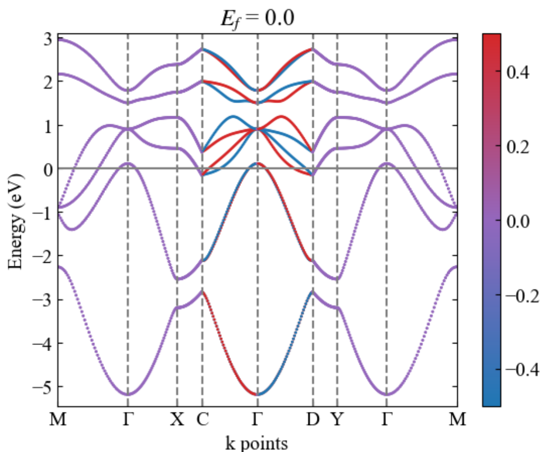
図 1.1: Cairo Pentagonal 構造の交替磁性 [2]
