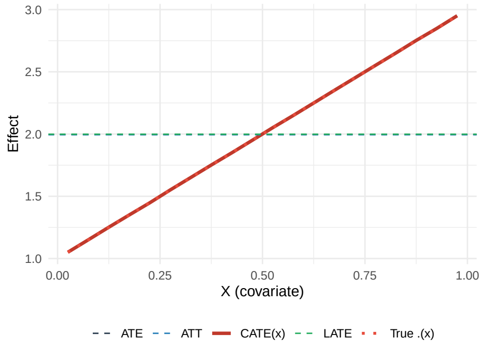
CATE(x) vs scalar estimands
