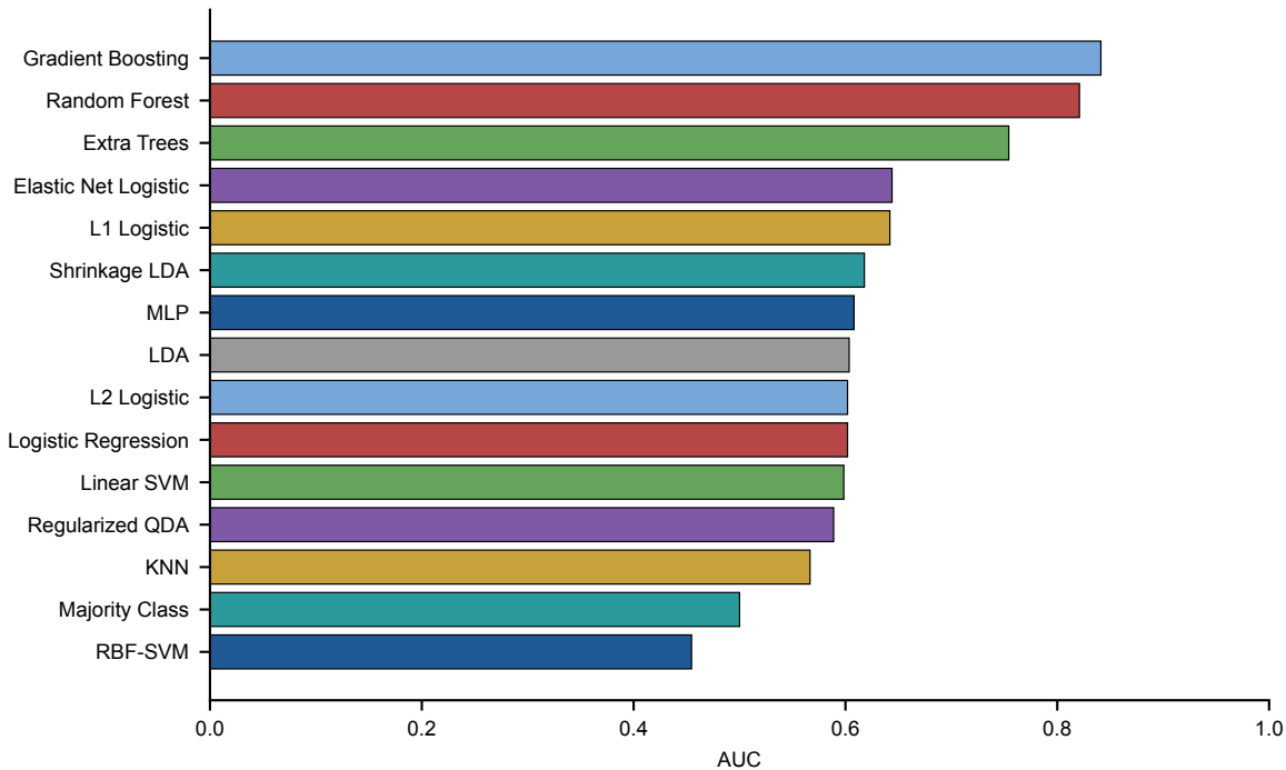
AUC comparison
