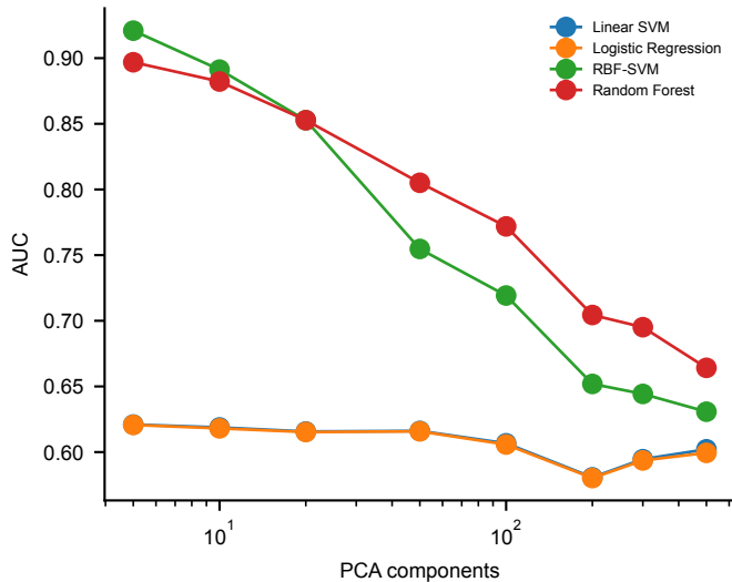
b PCA dimension vs AUC
