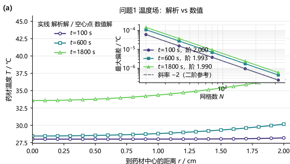
图1 问题1的解析对拍（回答”可靠性如何证明”）：代表时刻（100/600/1800 s）径向温度剖面，圆柱 Robin 特征展开解析解（线）vs 守恒有限体积数值解（点）；单元中心逐点最大偏差 5.9 \times 10^{-7} \text{ °C} ( N=320 )，插图为偏差随网格的收敛（实测阶 2.00）。两种完全不同的数学结构互证，排除离散、边界与时间积分错误。
