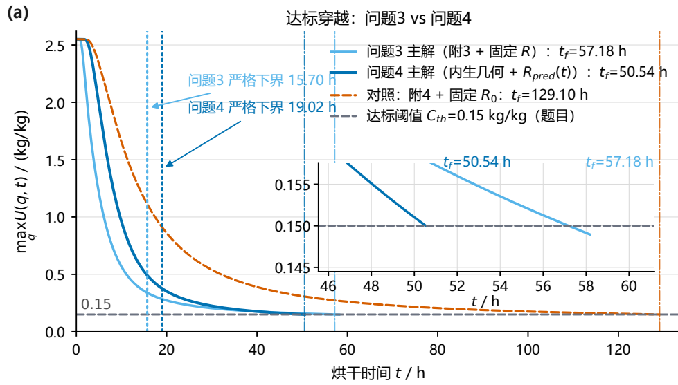
图4 达标穿越（回答“ t_f 多少、收缩贡献多大”）： \max_q U(q, t) 全程曲线与 0.15 阈值线；问题3 主解（ t_f = 57.1799 h）、问题4 主解（ t_f = 50.5369 h，内生几何）与附录4 固定半径对照（129.1047 h）三线对比，横轴标出复算严格下界（15.70 h / 19.02 h，低于此必错）。一图同时交付归因、判据与下界闸门。
