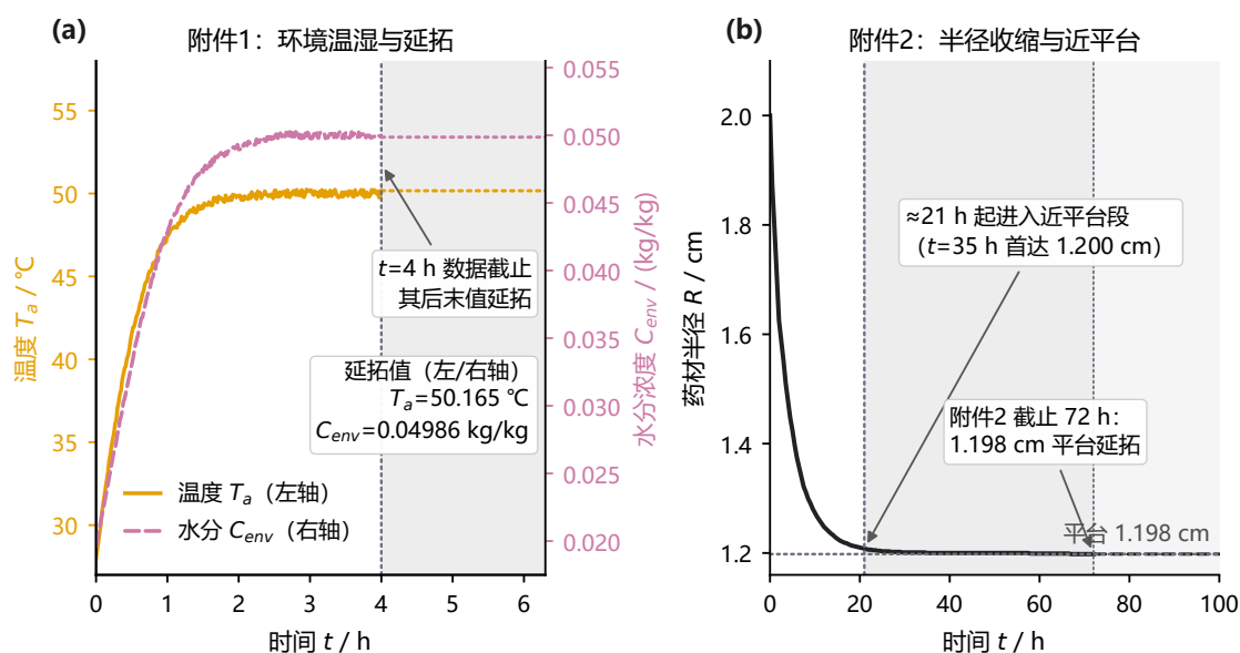
图2 输入数据与口径（回答”数据可用性如何裁定”）：附件1的温度与空气水分浓度（241点、60 s步、终于4 h；标出4 h截止与末值保持延拓 T_a = 50.165 \text{ °C} 、 C_{env} = 0.04986 ）；附件2外半径（145点、1800 s步，2.000→1.198 cm；标出约21 h进入近平台段）。读法：附件1只覆盖前4 h（需外推）；附件2覆盖0–72 h， t_f 仍在观测区间内。
