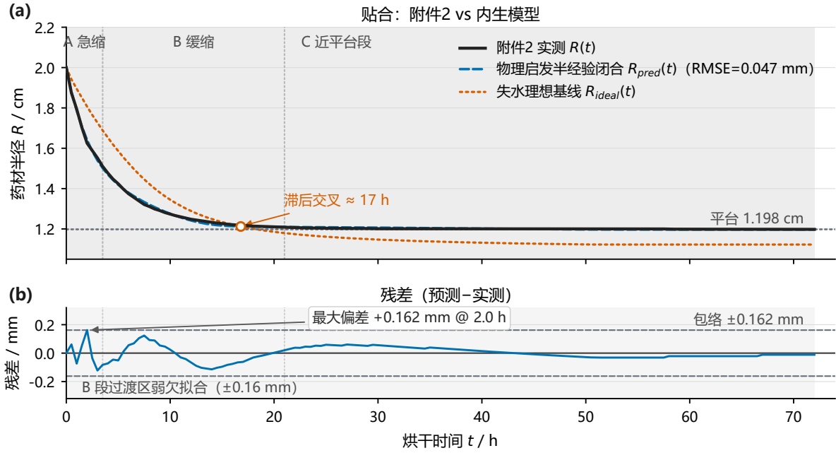
图 9 内生收缩模型对附件 2 的吻合与验证：式 (5.4) 由三项物理机制叠加而成，含 5 个标定参数与 2 个不参与拟合的量，它复现了附件 2 的全程形态：RMSE 0.047 mm，约为量化分辨率的 5 倍；滞后交叉 17.0 h，数据约 16 h；平台 1.1969 cm，数据 1.198 cm；三段形态全部复现。残差子图显示偏差始终在 \pm 0.16 mm 以内，这是以实测几何单向驱动得到的拟合指标
