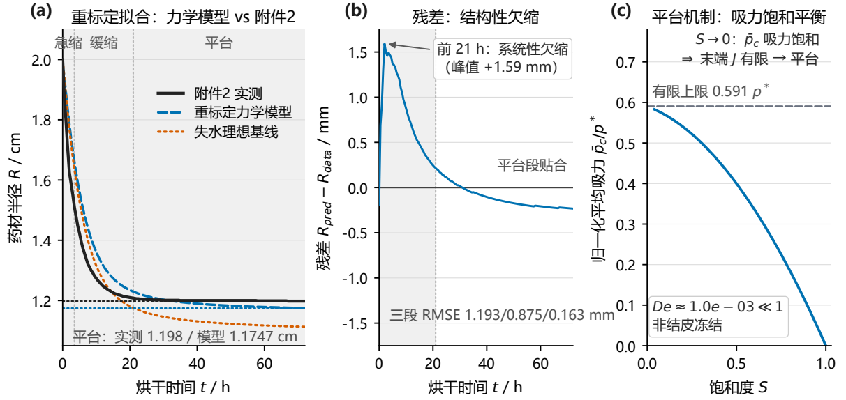
图 12 力学驱动内生收缩模型：修正后的数值格式与幂律保水重标定 ( \beta = 0.106 ) 对附件 2 的拟合结果为 RMSE 0.522 mm，残差在三段上分别为急缩 1.193、缓缩 0.875、平台 0.163 mm， t_f = 51.1667 h；末端 60–72 h 仅再降 0.04 mm，已真正进入平台，平台机制为吸力饱和平衡，此时 De \approx 10^{-3} \ll 1 。(c) 面板给出该平台机制：归一化平均吸力 \bar{p}_c/p^* 随饱和度 S 下降而单调上升，并在 S \rightarrow 0 时趋于有限上限 p^*/[(1-\beta)(2-\beta)] ，末端收缩进入平台即来自这一吸力饱和平衡；气相体积份额全程非负， g_{\min} = 0.1446 ，见表 3
