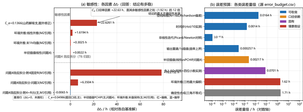
图 5 敏感性条形图（回答”结论有多稳”）：各因素 \Delta t_f 横向条形， C_e 长条自然主导——诚实展示最大不确定性来源。
