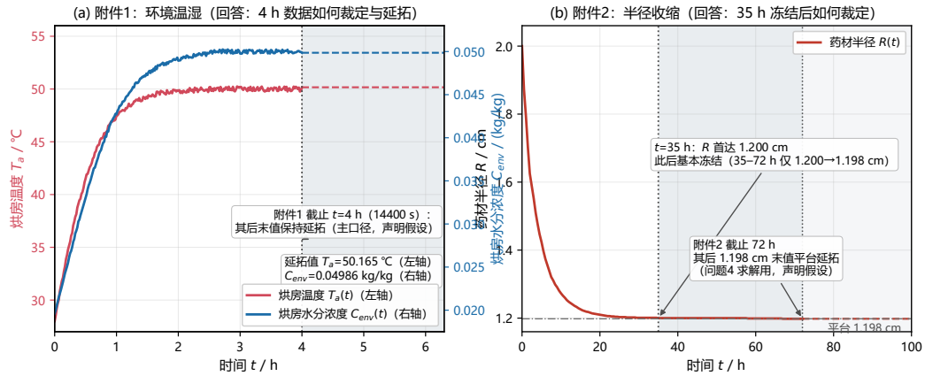
图 2 输入数据与口径（回答“数据可用性如何裁定”）：附件 1 的温度与空气水分浓度（标出 4 h 截止与末值保持延拓）；附件 2 外半径（标出 35 h 冻结与平台延拓）。
