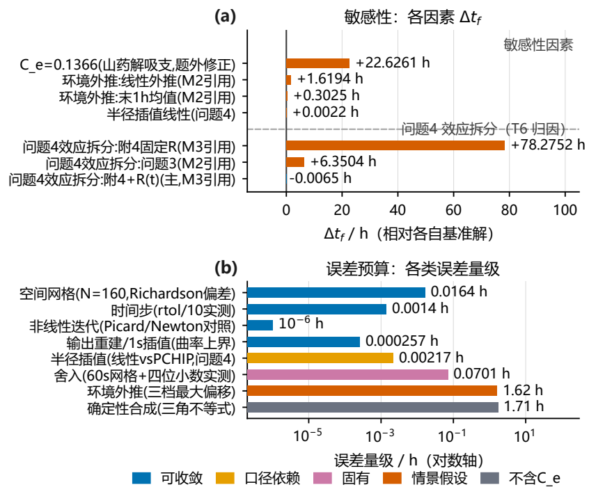
图 7 敏感性条形图（回答“结论有多稳”）：各因素 \Delta t_f 横向条形——边界汇口径 C_e = 0.1366 （题外修正）+22.63 h 自然主导，环境外推 +1.62 h 次之，半径插值仅 +0.002 h；诚实展示最大不确定性来源，主结果一律用题目口径。
