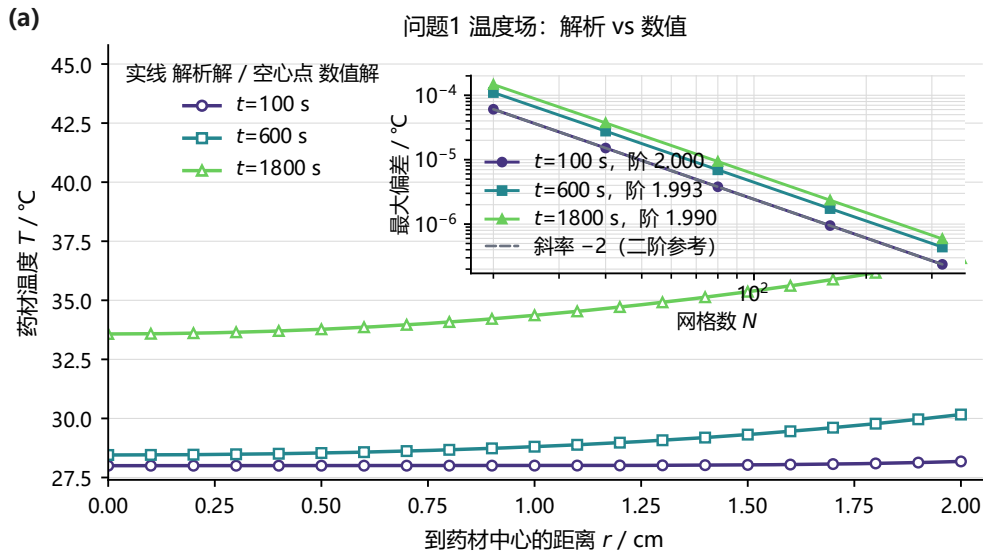
图 1 问题 1 的解析对拍（回答“可靠性如何证明”）：代表时刻（100/600/1800 s）径向温度剖面，圆柱 Robin 特征展开解析解（线）vs 守恒有限体积数值解（点）；单元中心逐点最大偏差 5.9 \times 10^{-7} \text{ }^{\circ}\text{C} ( N=320 )，插图为偏差随网格的收敛（实测阶 2.00）。两种完全不同的数学结构互证，排除离散、边界与时间积分错误。
