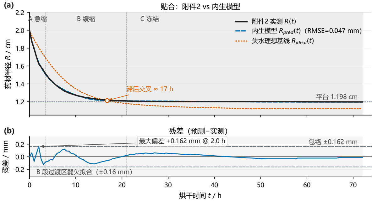
图 5 内生收缩模型对附件 2 的贴合与验证（回答“收缩能否由模型内生预测”）：三项第一性原理机制叠加的闭合（式 (6.1)，5 个标定参数 + 2 个文献量）几乎完美复现附件 2——RMSE 0.047 mm（量化分辨率的 5 倍）、滞后交叉（17.0 h vs 约 16 h）、平台（1.1969 vs 1.198 cm）、三段形态全对；残差子图显示偏差有界在 \pm 0.16 mm。
