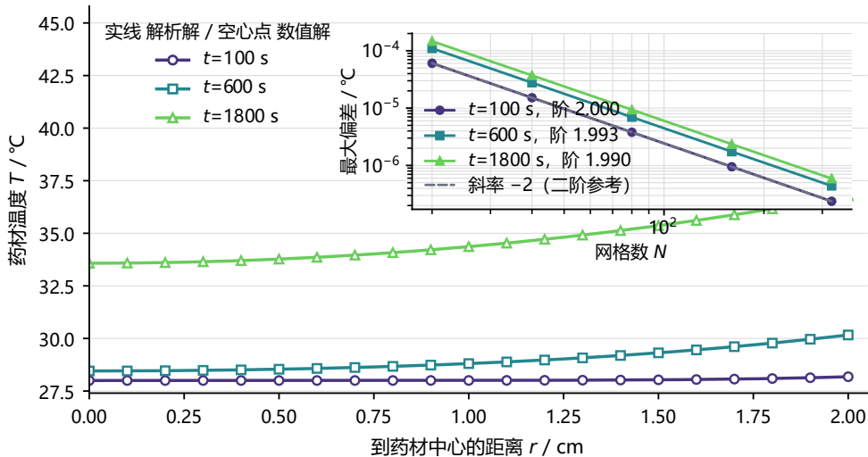
(a) 问题1 温度场：解析 vs 数值
