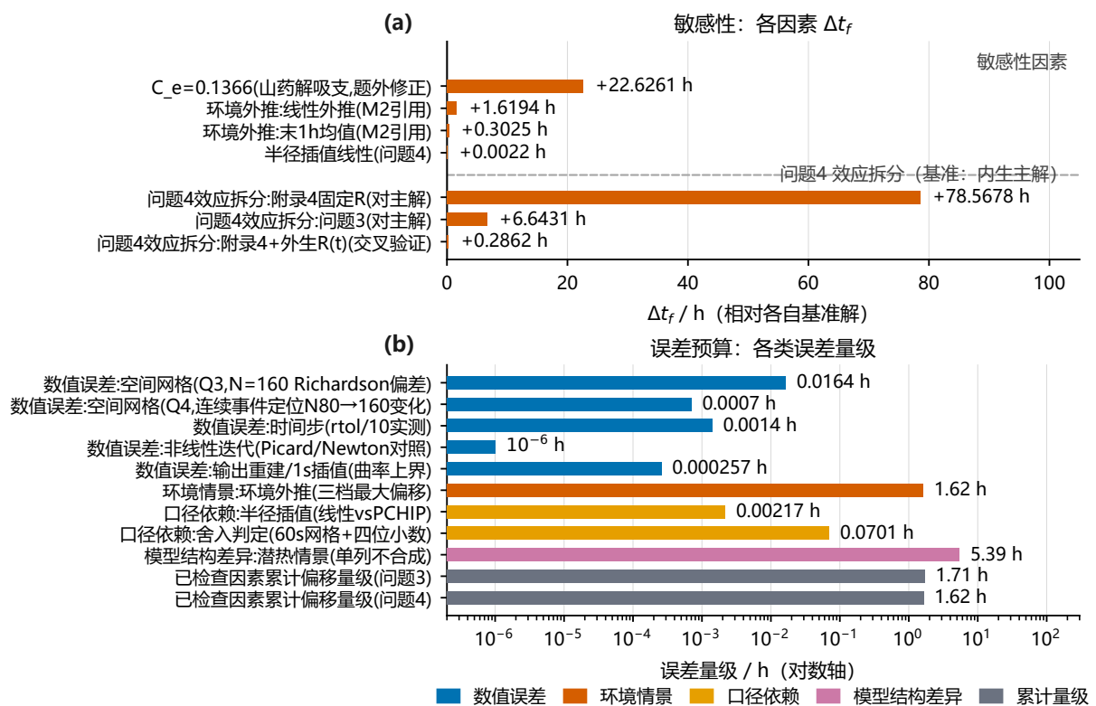
图 10 敏感性条形图(回答“结论有多稳”): 各因素 \Delta t_f 横向条形——边界汇口径 C_e = 0.1366 (题外修正) +22.63 h 自然主导, 环境外推 +1.62 h 次之, 半径插值仅 +0.002 h; 诚实展示最大不确定性来源, 主结果一律用声明闭合口径。
