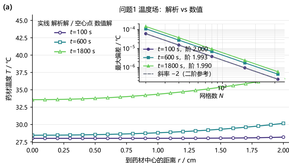
图 1 问题 1 的解析对拍（回答“可靠性如何证明”）：代表时刻（100/600/1800 s）径向温度剖面，圆柱 Robin 特征展开解析解（线）vs 守恒有限体积数值解（点）；单元中心逐点最大偏差 5.9 \times 10^{-7} ^\circ\text{C} ( N=320 )，插图为偏差随网格的收敛（实测阶 2.00）。两种完全不同的数学结构互证，排除离散、边界与时间积分错误。
