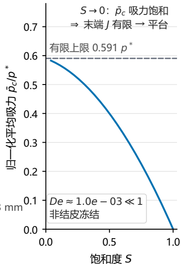
(c) 平台机制：吸力饱和平衡
