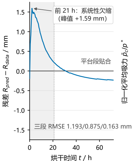
(b) 残差：结构性欠缩
