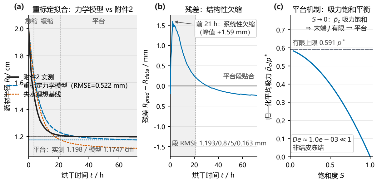
图 9 力学驱动内生收缩模型（回答”半径能否由材料变形求出”）：(a) 求解器（热算子经独立退化对拍验证）+ 幂律保水重标定（ \beta = 0.106 ）对附件 2 的拟合——RMSE 0.522 mm（残差三段：急缩 1.193 / 缓缩 0.875 / 平台 0.163 mm）、 t_f = 51.1667 h；末端 60–72 h 仅再降 0.04 mm（真平台）。(b) 残差 R_{pred} - R_{data} 随时间：0–21 h 系统性欠缩（峰值 +1.59 mm @ 2 h），平台段贴合。(c) 平台机制为吸力饱和平衡：归一化平均吸力在 S \rightarrow 0 时饱和于有限上限 0.591 p^* （该上限由标定 \beta 定），故末端 J 有限、半径停止收缩；标定参数下表面 De \approx 10^{-3} \ll 1 ，非黏弹冻结。
