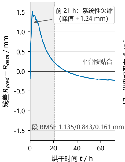
(b) 残差：结构性欠缩
